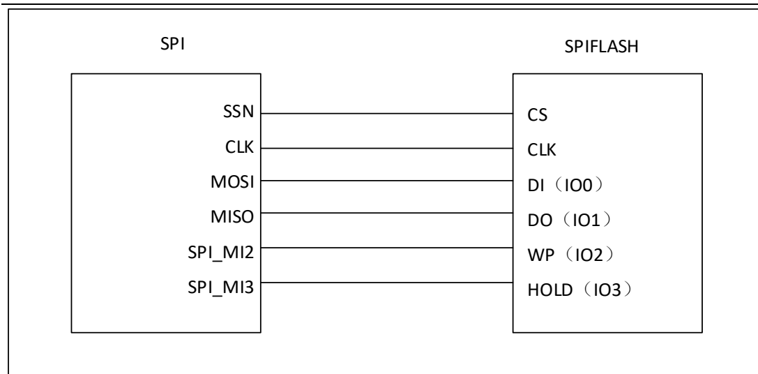
图 6-56 SPIFLASH 四线模式外部连接图
