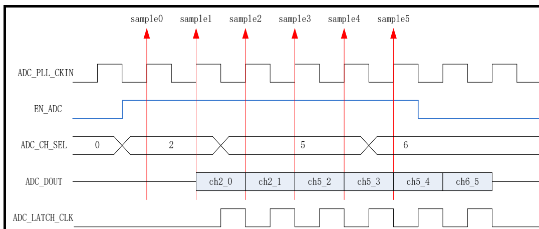
图 6-83 SAR ADC 多通道连续采样示意图
