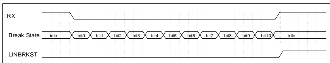
图 6-41 Break 信号足够长示意图
