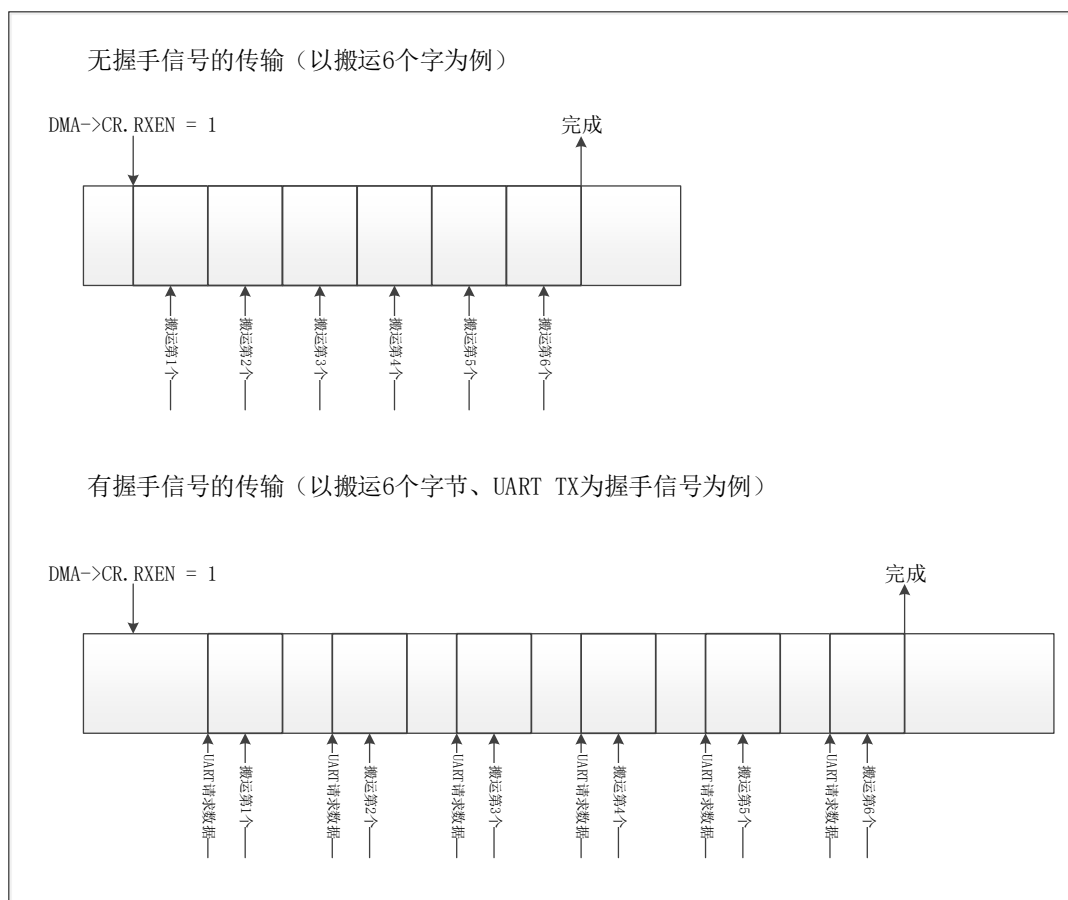
图 6-86 握手、非握手信号传输图
