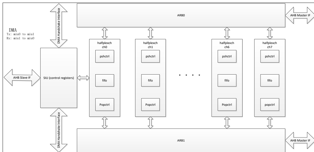
图 6-84 DMA 模块结构图
