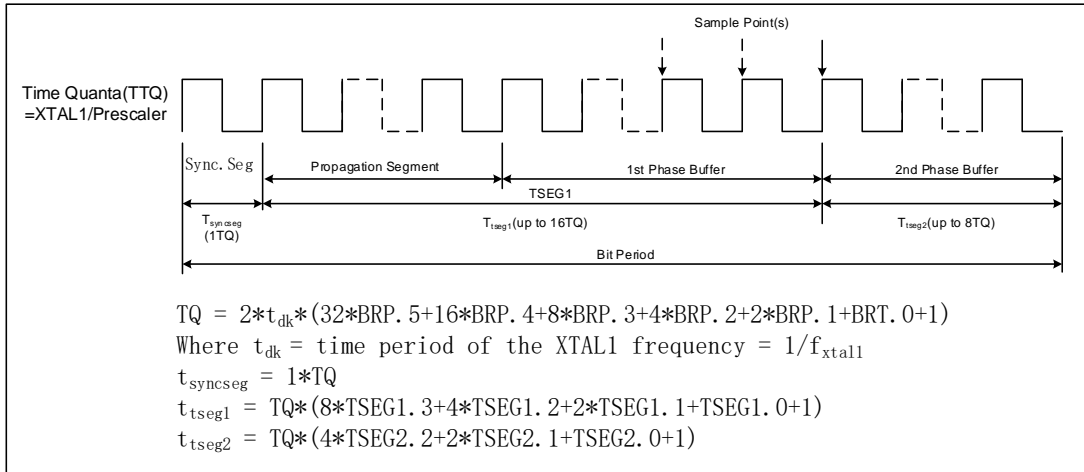
图 6-88 波特率设置示意图
