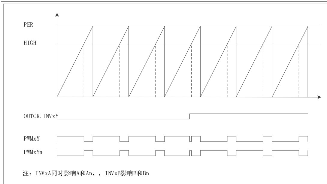
图 6-76 电平翻转示意图
