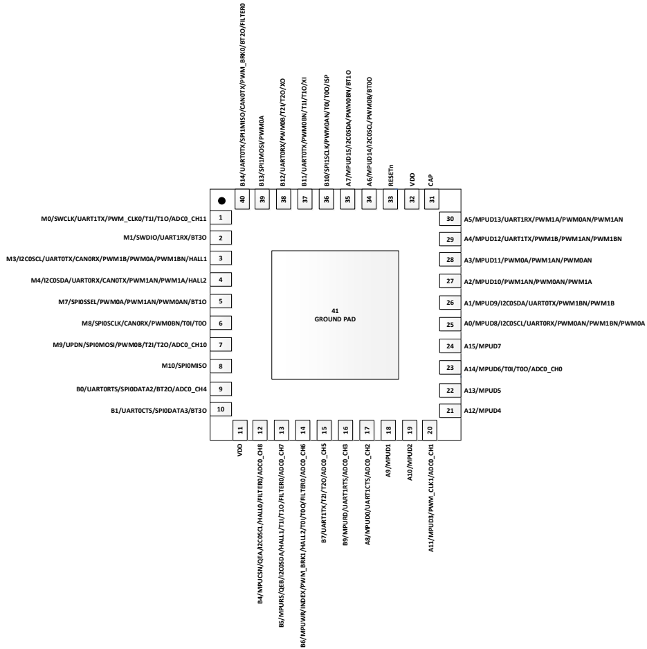
图 5-1 SWM166D8U6 封装管脚配置图
