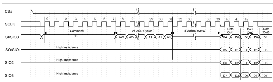
图 6-55 SPIFLASH 四线读帧格式
