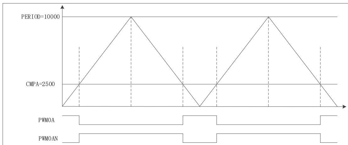
图 6-77 挖坑前波形
