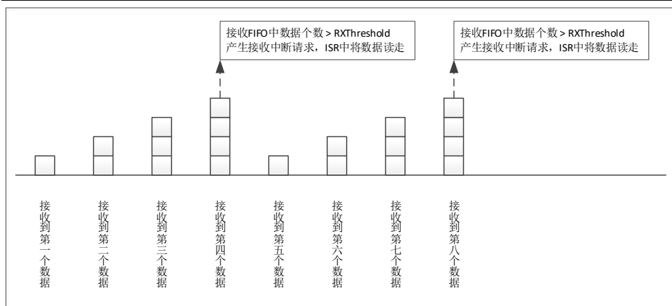
图 6-43 对方发送 8 个数据接收 FIFO 示意图
