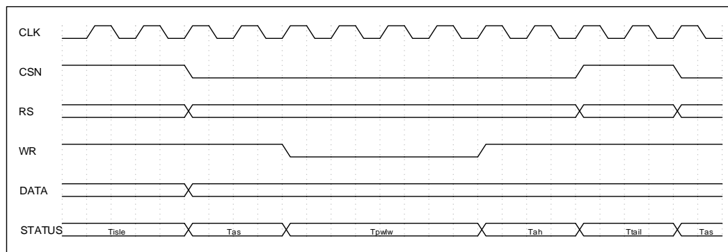
图 6-90 MPU 接口时序图
