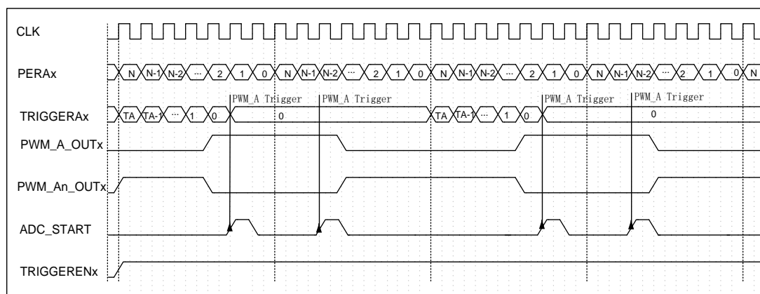
图 6-81 中心对称模式下 PWM 触发 ADC 采样示意图
