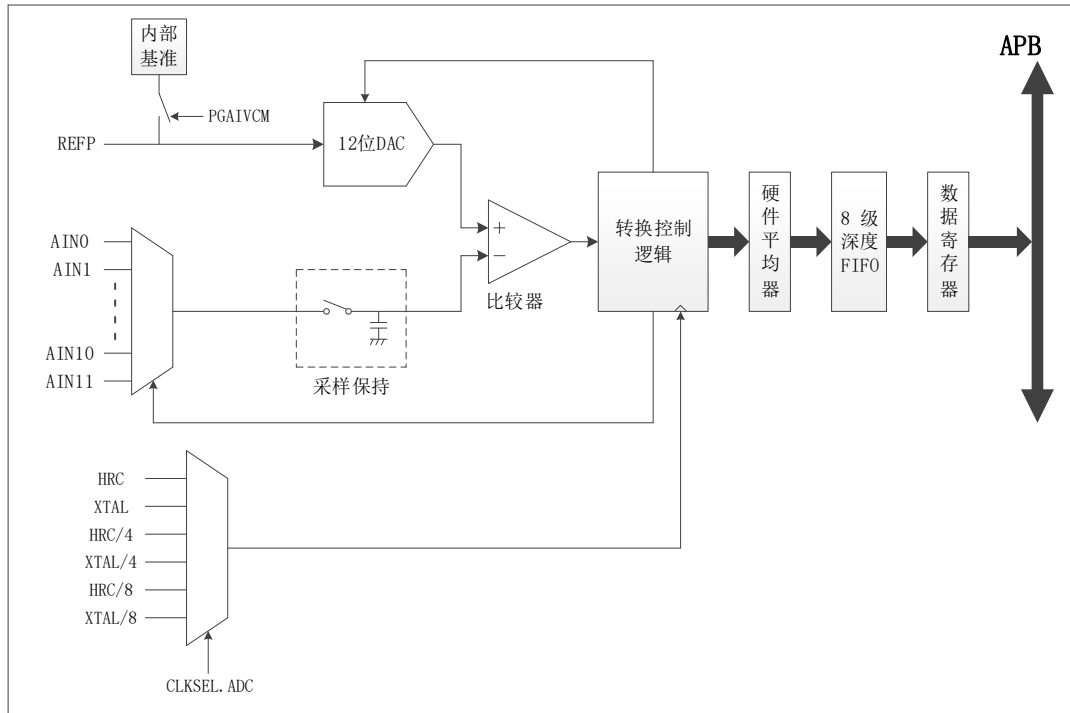
图 6-79 ADC 模块结构框图
