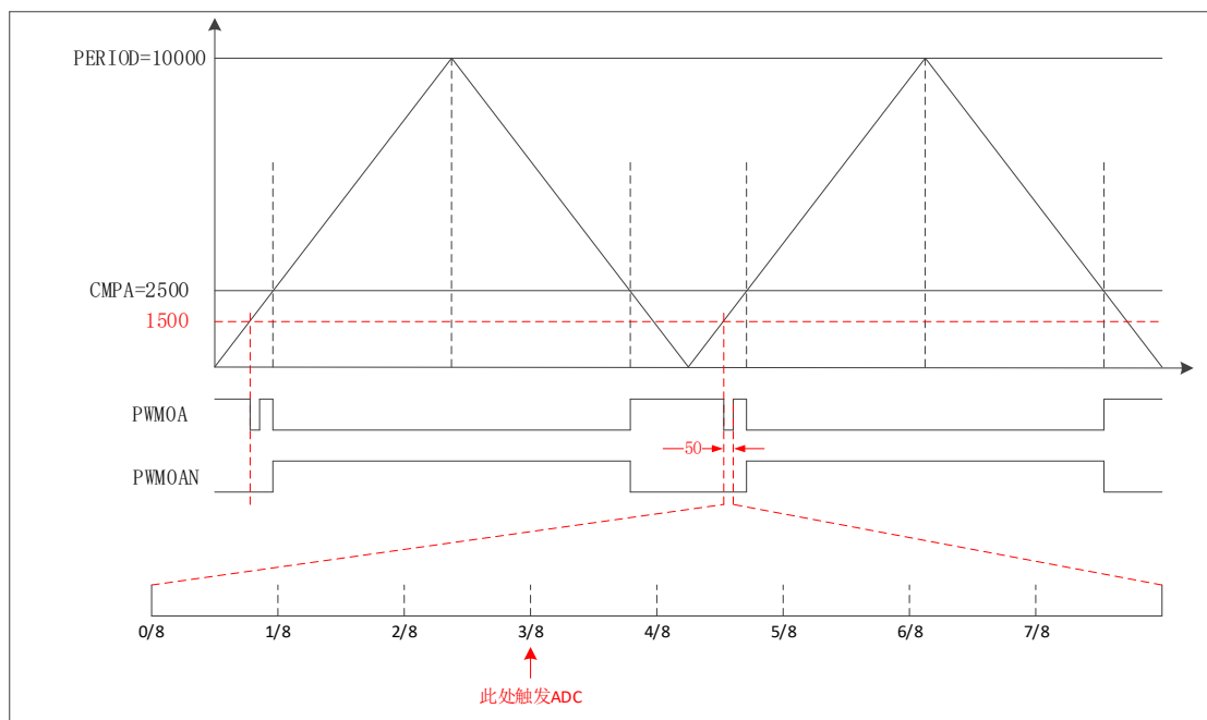
图 6-78 挖坑后波形
