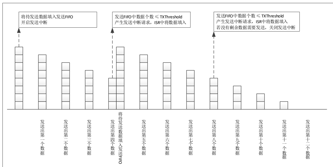
图 6-45 发送 FIFO 示意图
