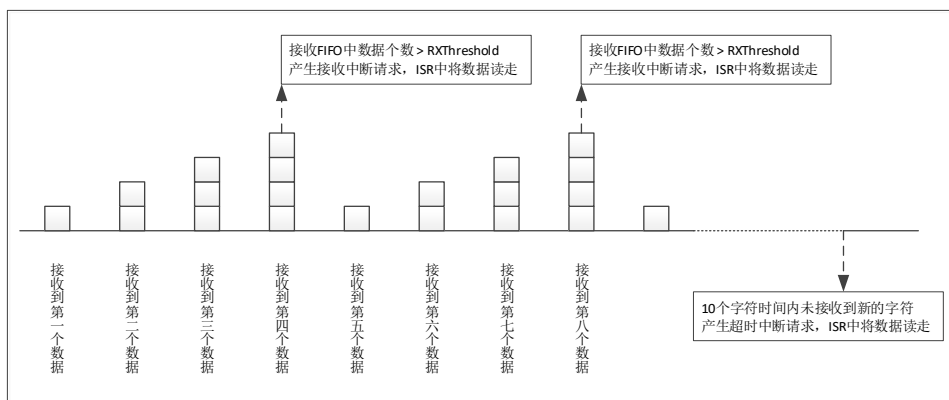
图 6-44 对方发送 9 个数据接收 FIFO 示意图
