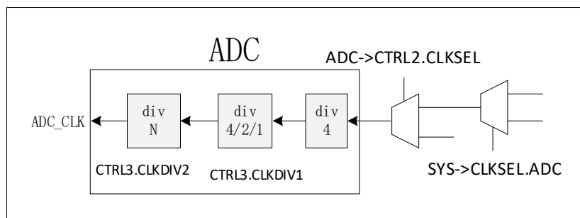
图 6-80 ADC 时钟示意图
