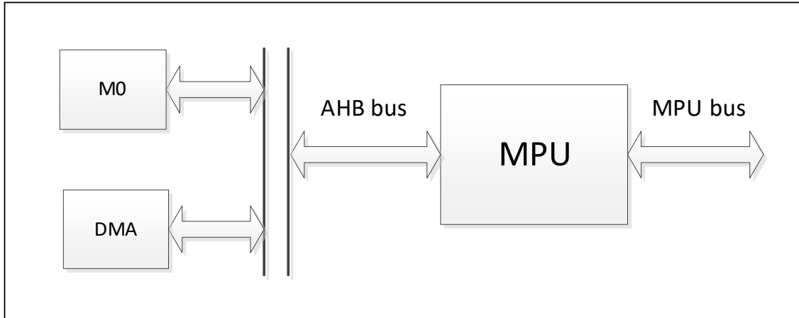
图 6-89 MPU 模块结构框图
