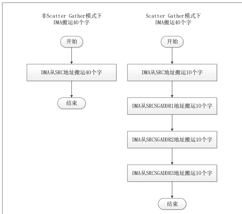
图 6-85 DMA 搬运 40 个字流程图
