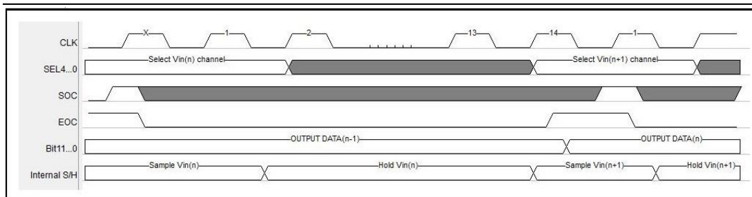
图 6-82 SAR ADC 连续采样示意图
