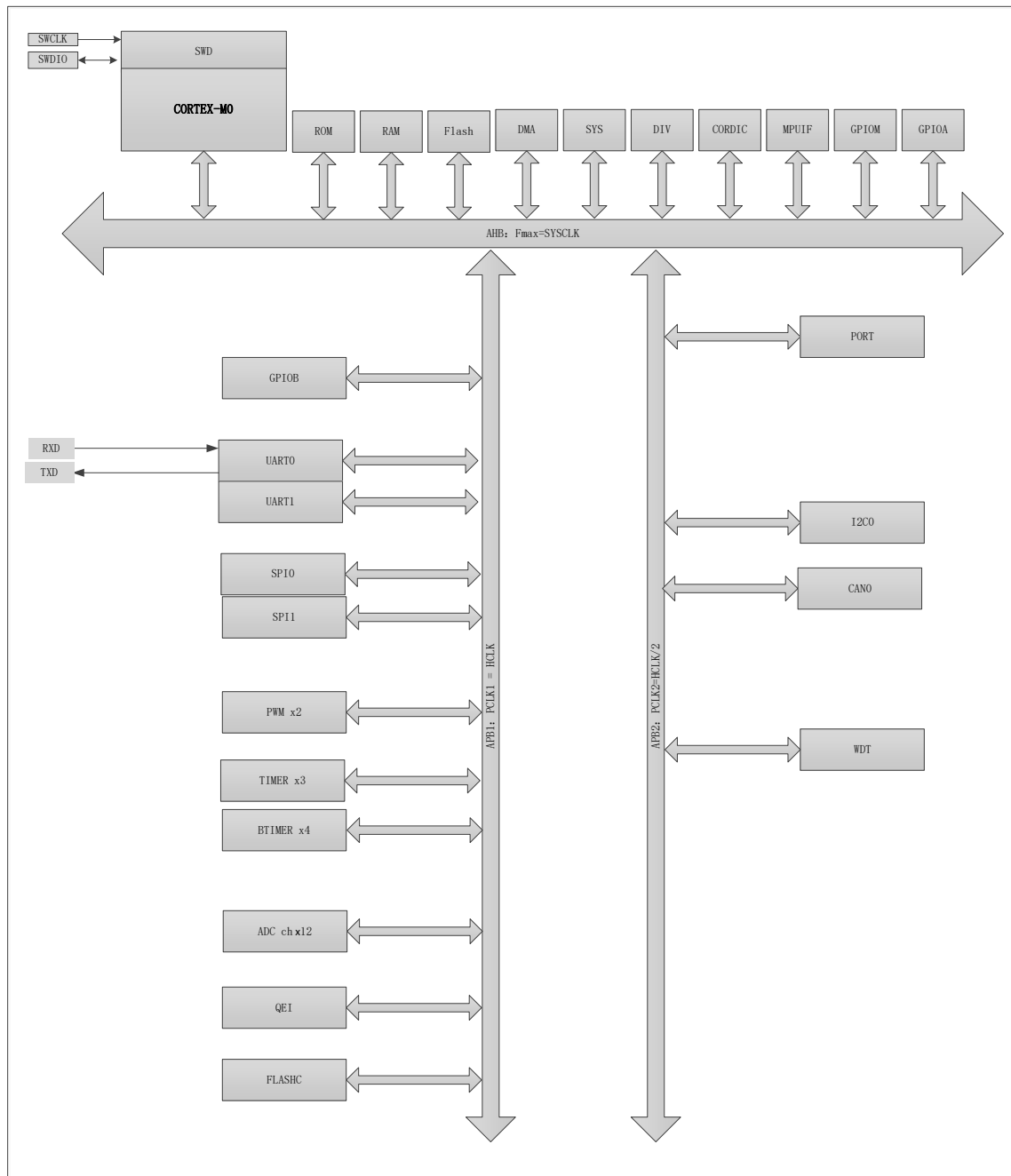
图 4-1 功能方框图
