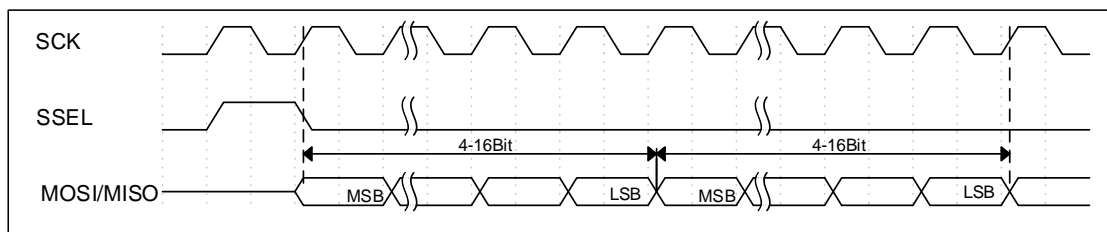
图 6-54 SSI 模式连续输出波形
