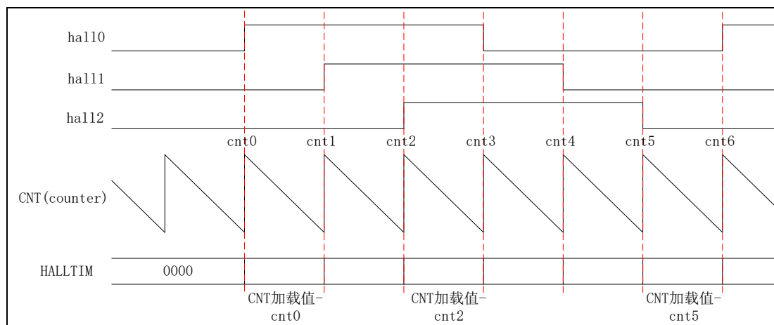
图 6-17 HALL 记录值
