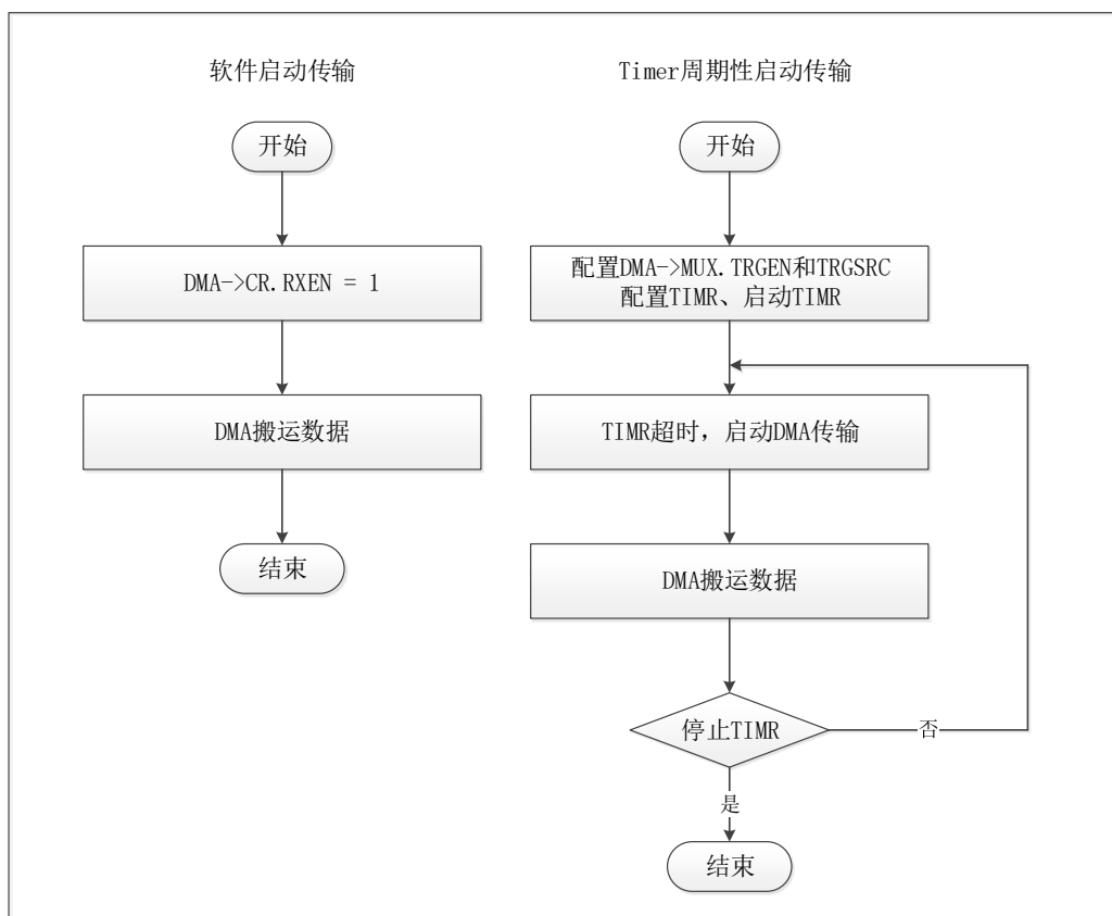
图 6-87 DMA 启动方式
