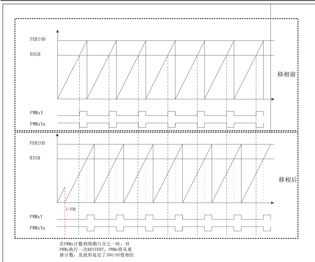
图 6-68 PWM 移相示意图
