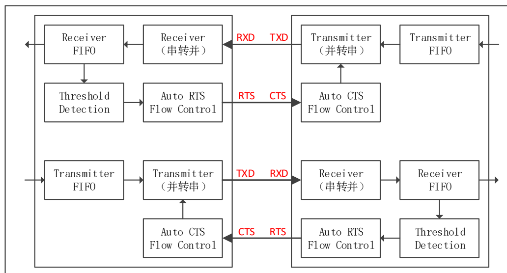
图 6-42 硬件流控
