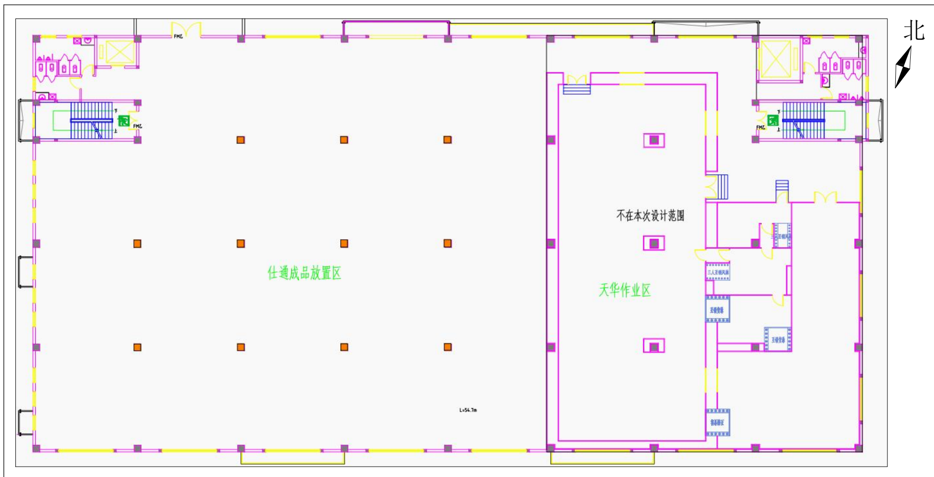
附图 4-5 北 2F 平面布置图
