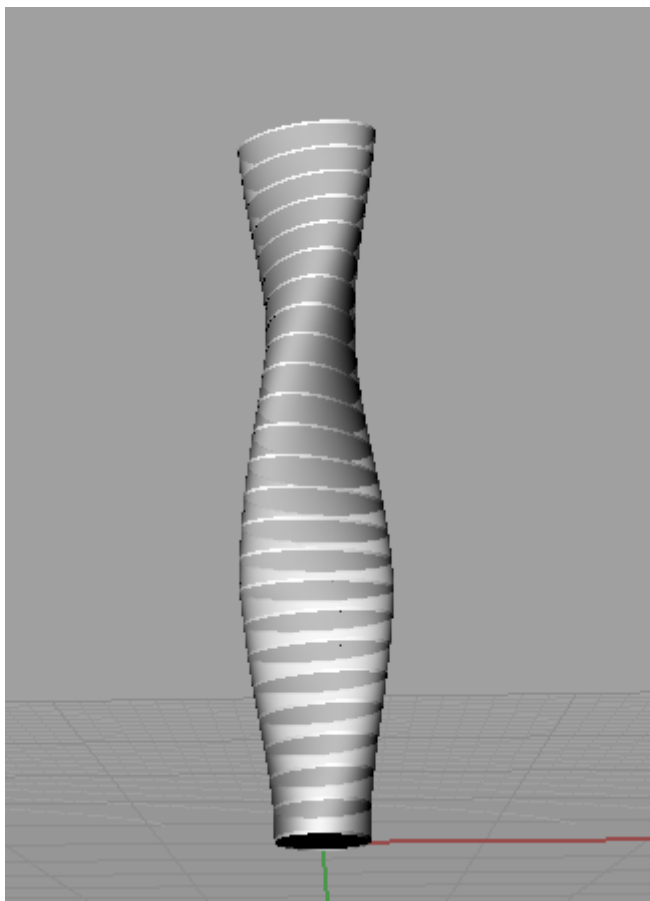
图 5.18: 最后效果。
