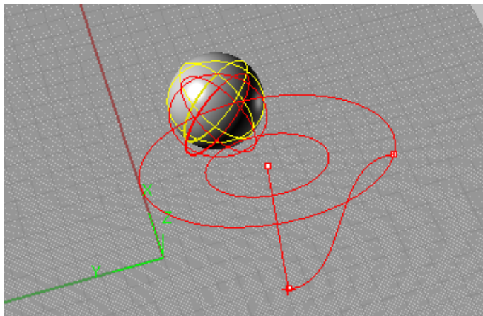
图 8.10: SOFTMOVE。
