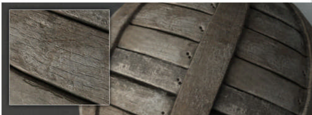
图 10.13: 置换贴图。
