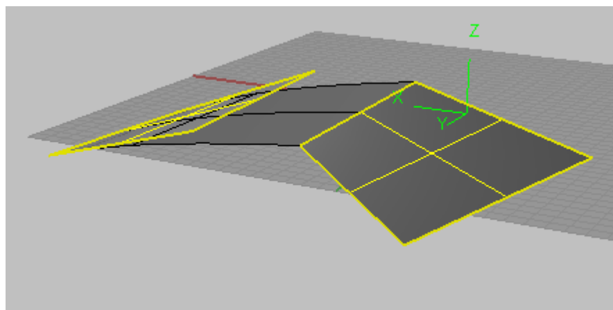
图 6.41: 位置连续。
