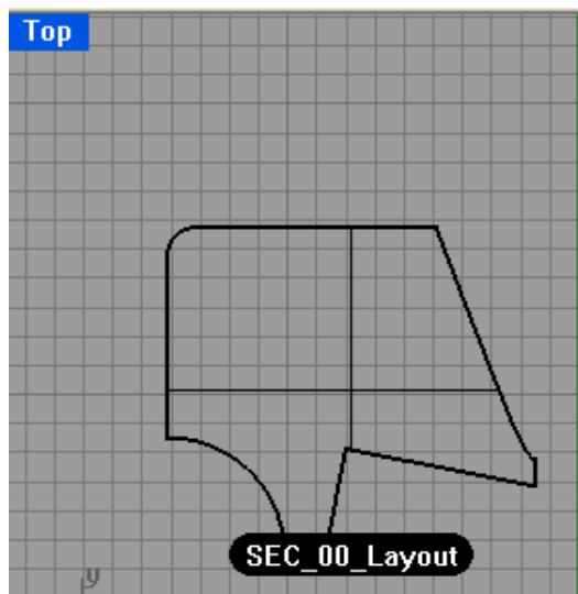
图 9.19: top 视图。
