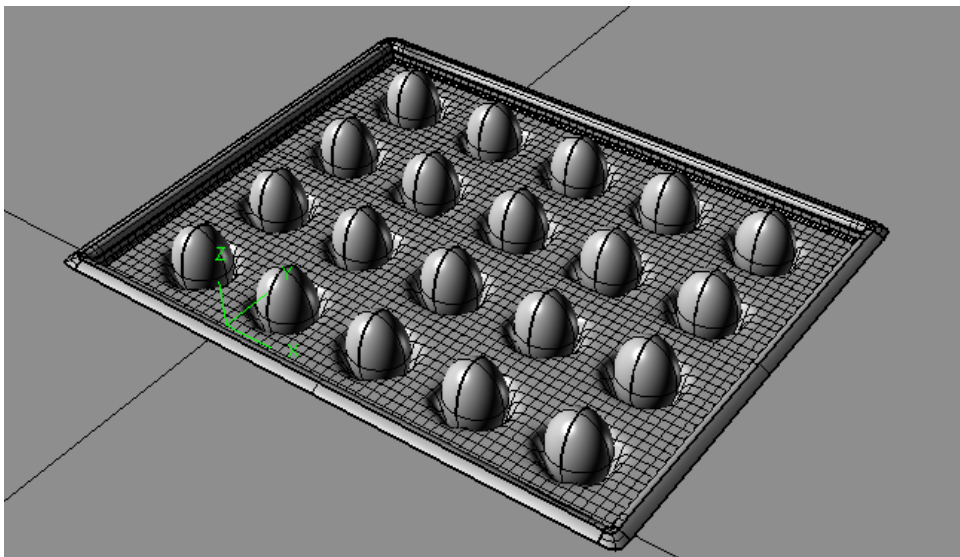
图 10.14：模型。
