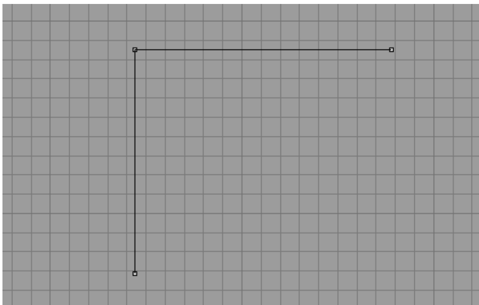
图 6.45: G0 连续。
