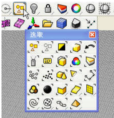
图 2.23: 选择工具集。
