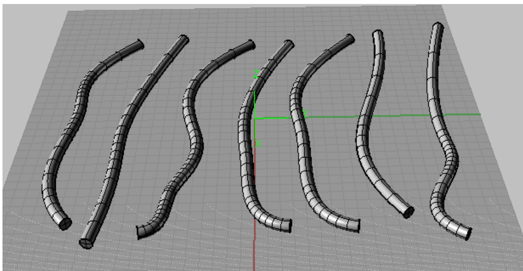
图 7.8：最终效果。
