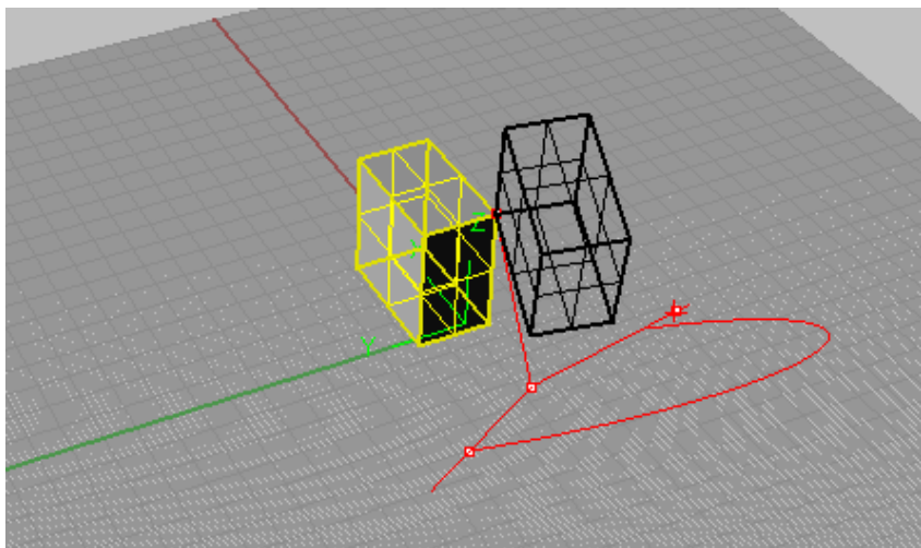
图 8.13: 3D 旋转。
