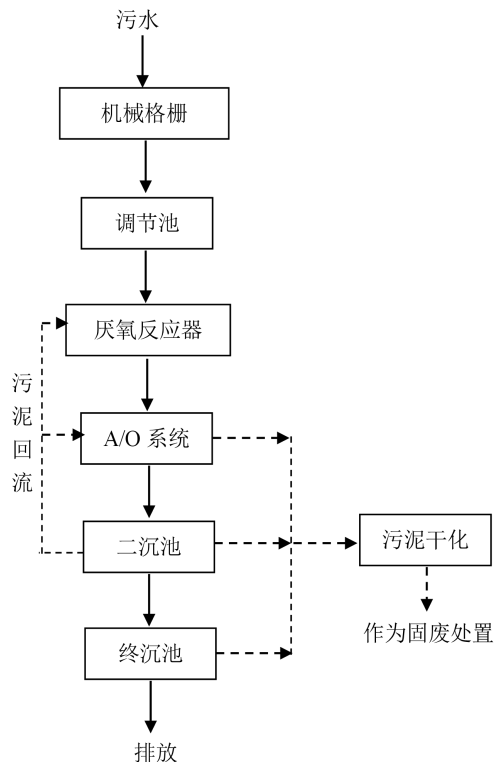
图4-2 污水处理站污水处理工艺流程图
