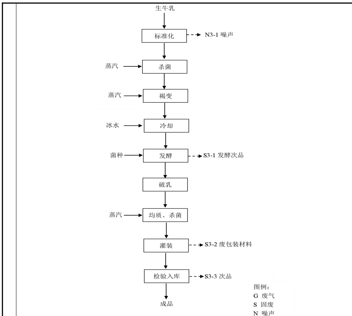
图 2-5 饮用型发酵乳生产工艺流程及产污节点示意图
