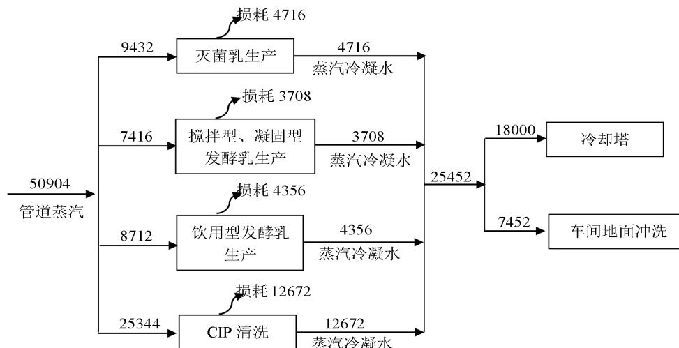
图 2-1 蒸汽平衡图（单位：t/a）
