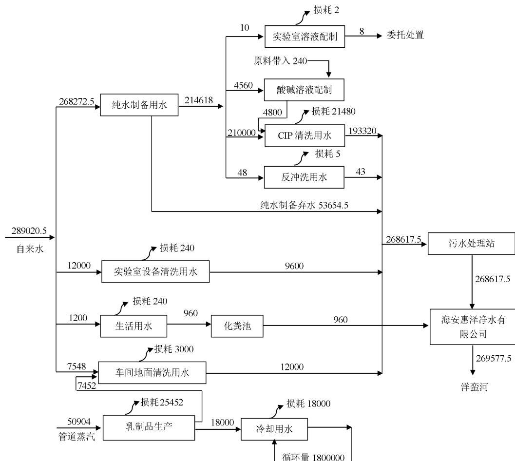
图 2-2 本项目水平衡图（单位：m 3 /a）
