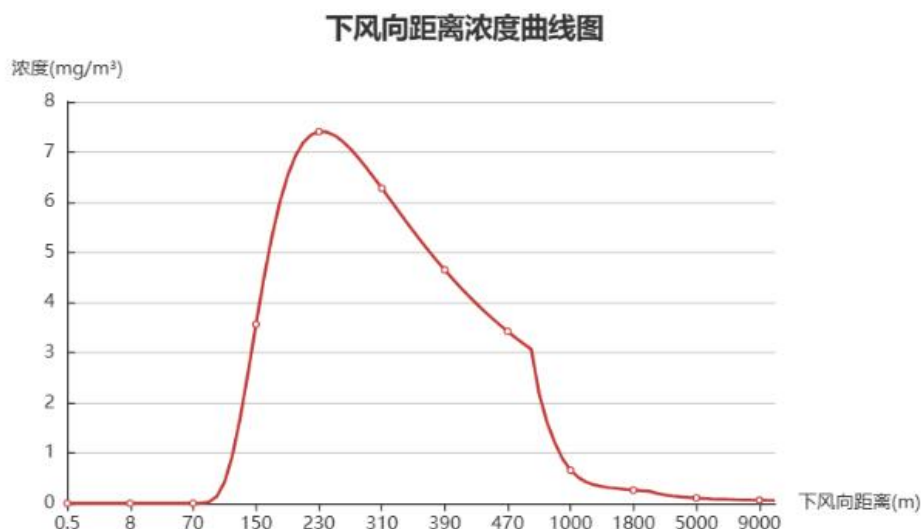
图 6.1-3 最不利气象条件 F 下 HCN 轴线最大浓度
