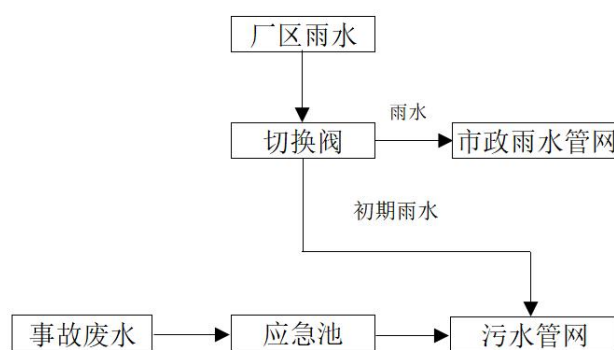
图 7.1-1 项目事故水收集系统
