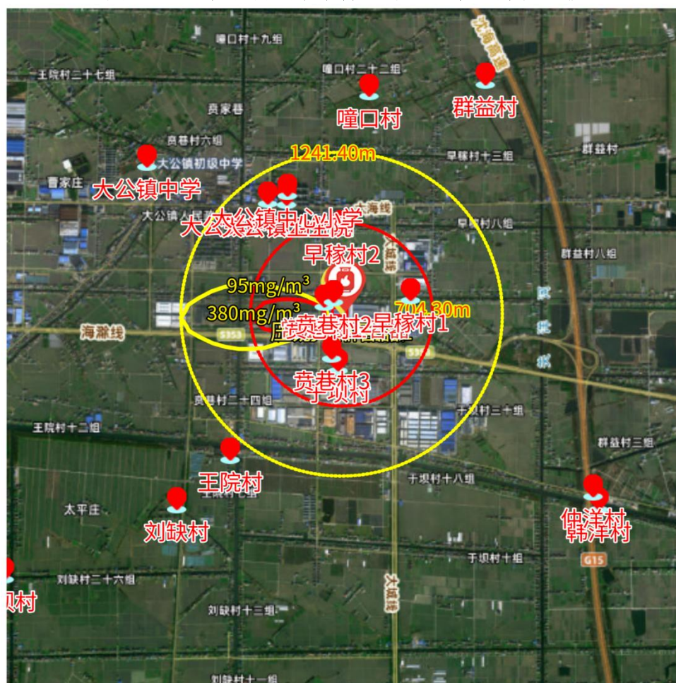
图 6.1-2 CO 浓度达到评价标准时的最大影响范围图
