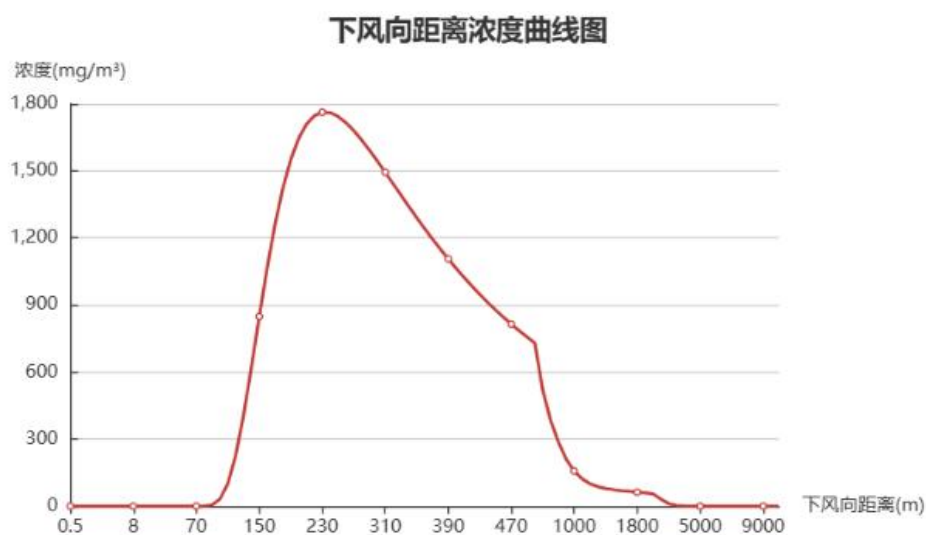
图 6.1-1 最不利气象条件 F 下 CO 轴线最大浓度
