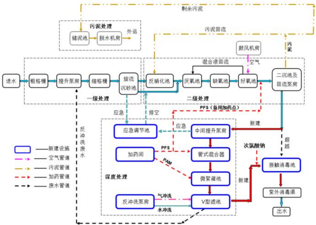
图 4-3 李堡滇池水务有限公司工艺流程图
