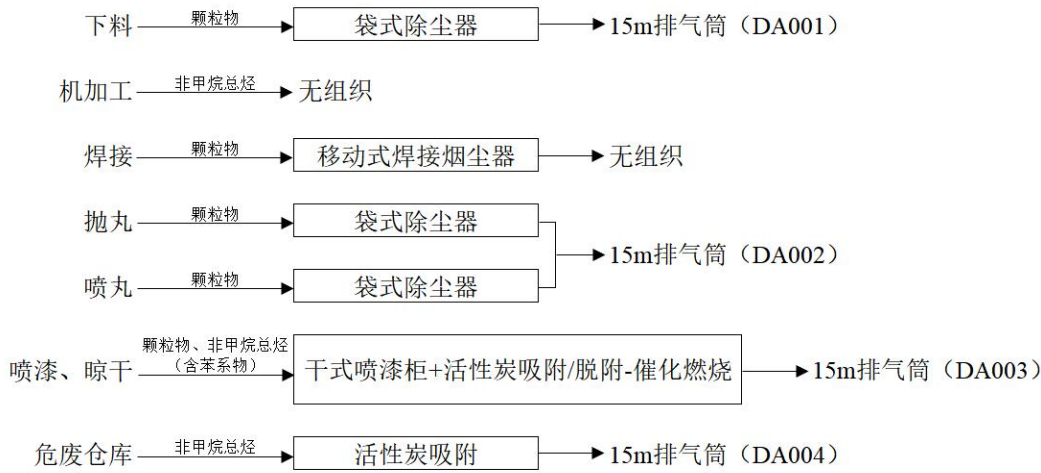
图 4-1 废气处置方式示意图
