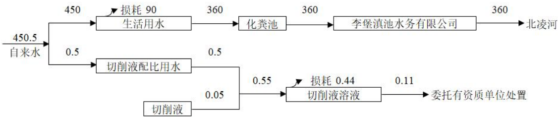
图 2-2 建设项目营运期水平衡图（单位：t/a）
