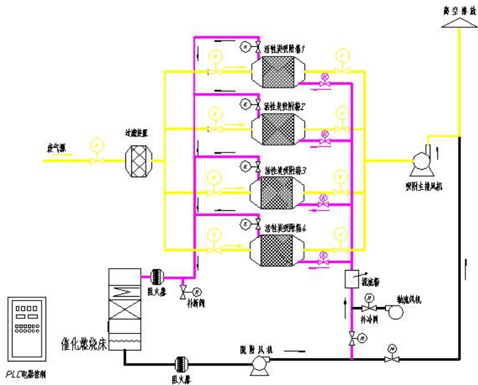
图 4-2 干式喷漆柜+活性炭吸附+脱附-催化燃烧示意图
