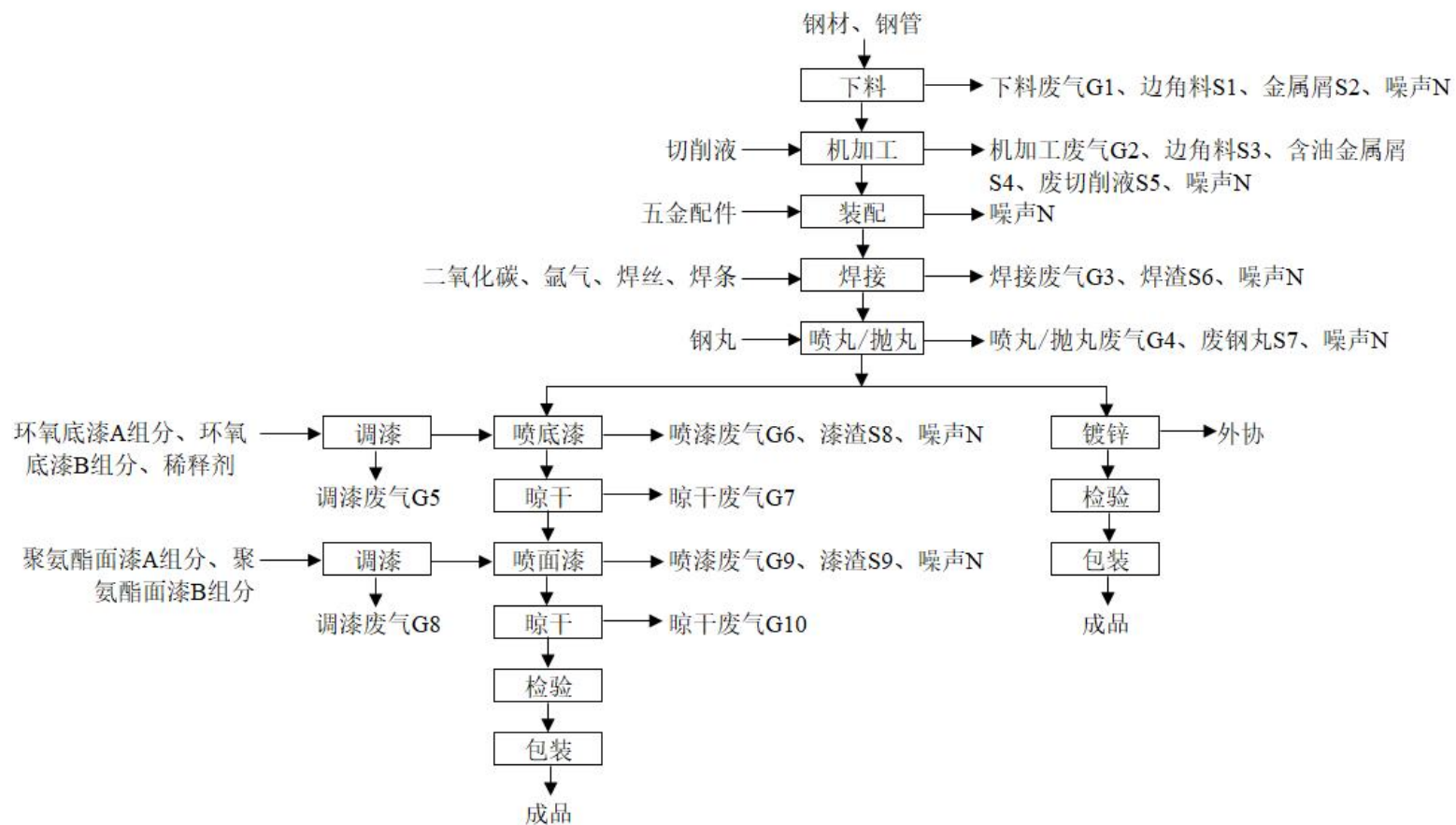
图 2-3 工艺流程图
