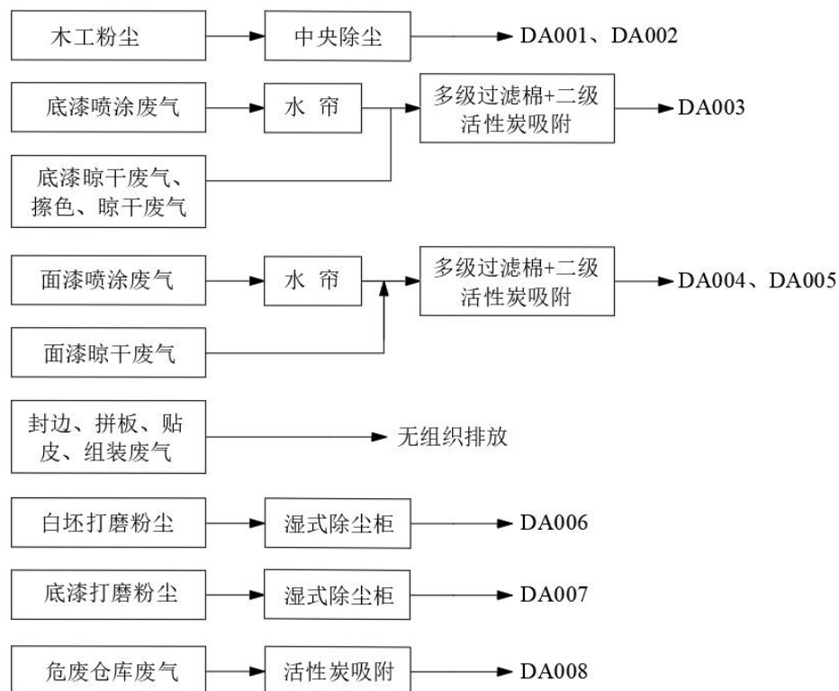
图 4-1 本项目废气收集、处理方式示意图
