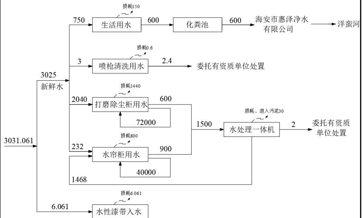
图 2-2 营运期水平衡图 (单位: t/a)
