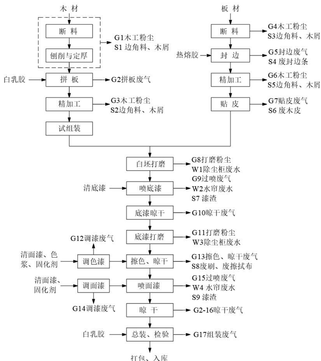
图 2-3 实木家具生产工艺流程及产污节点示意图
