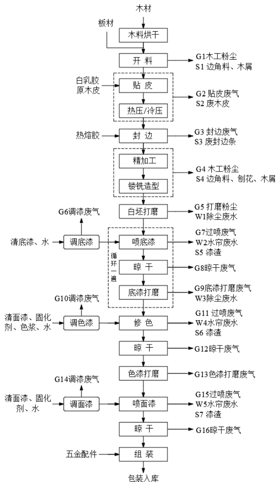
图 2-3 生产工艺流程及产污节点示意图
