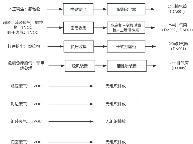
图 4-1 建设项目废气收集、处置方式示意图
