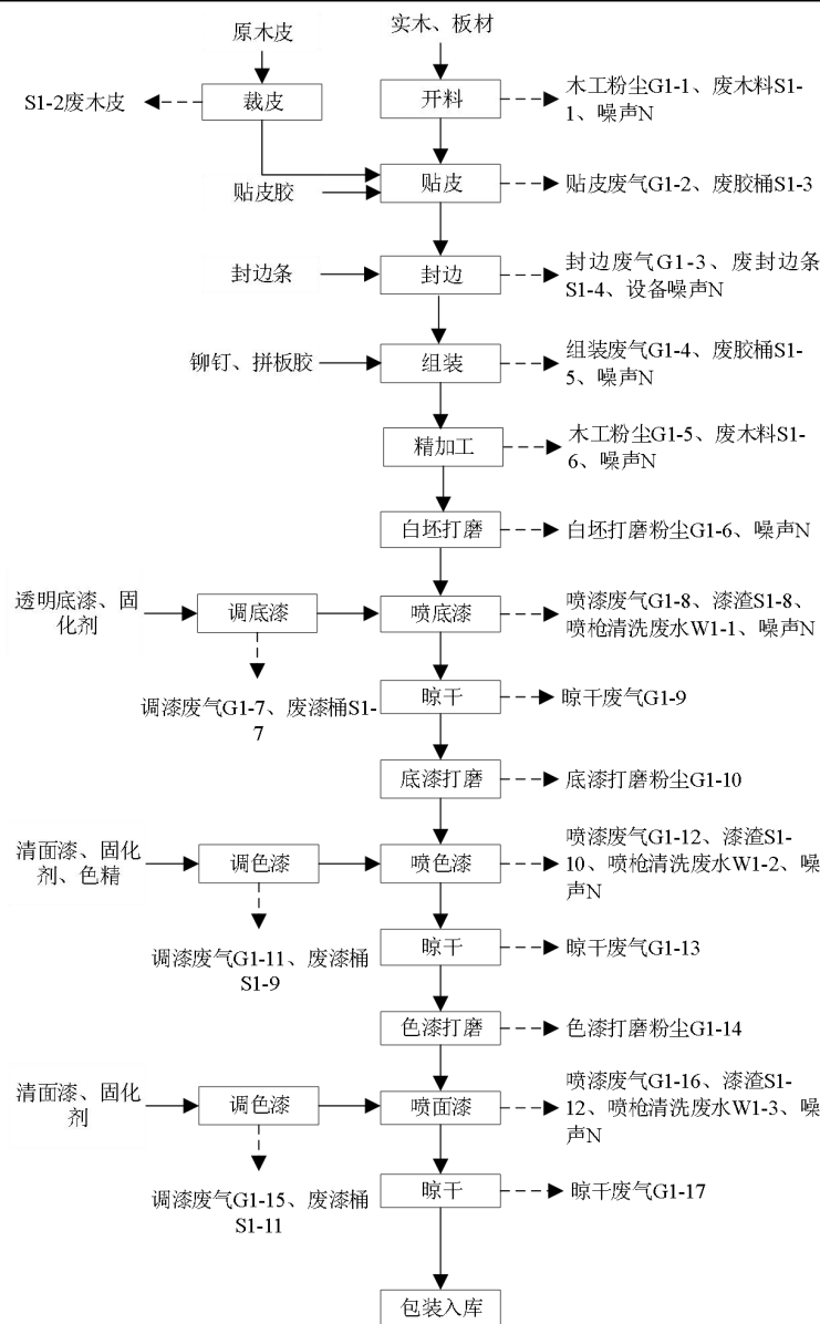
图 2-7 酒店喷漆家具工艺流程及产污环节图
