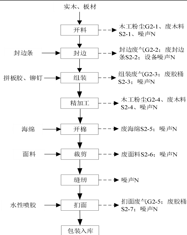
图 2-7 酒店软包家具工艺流程及产污环节图
