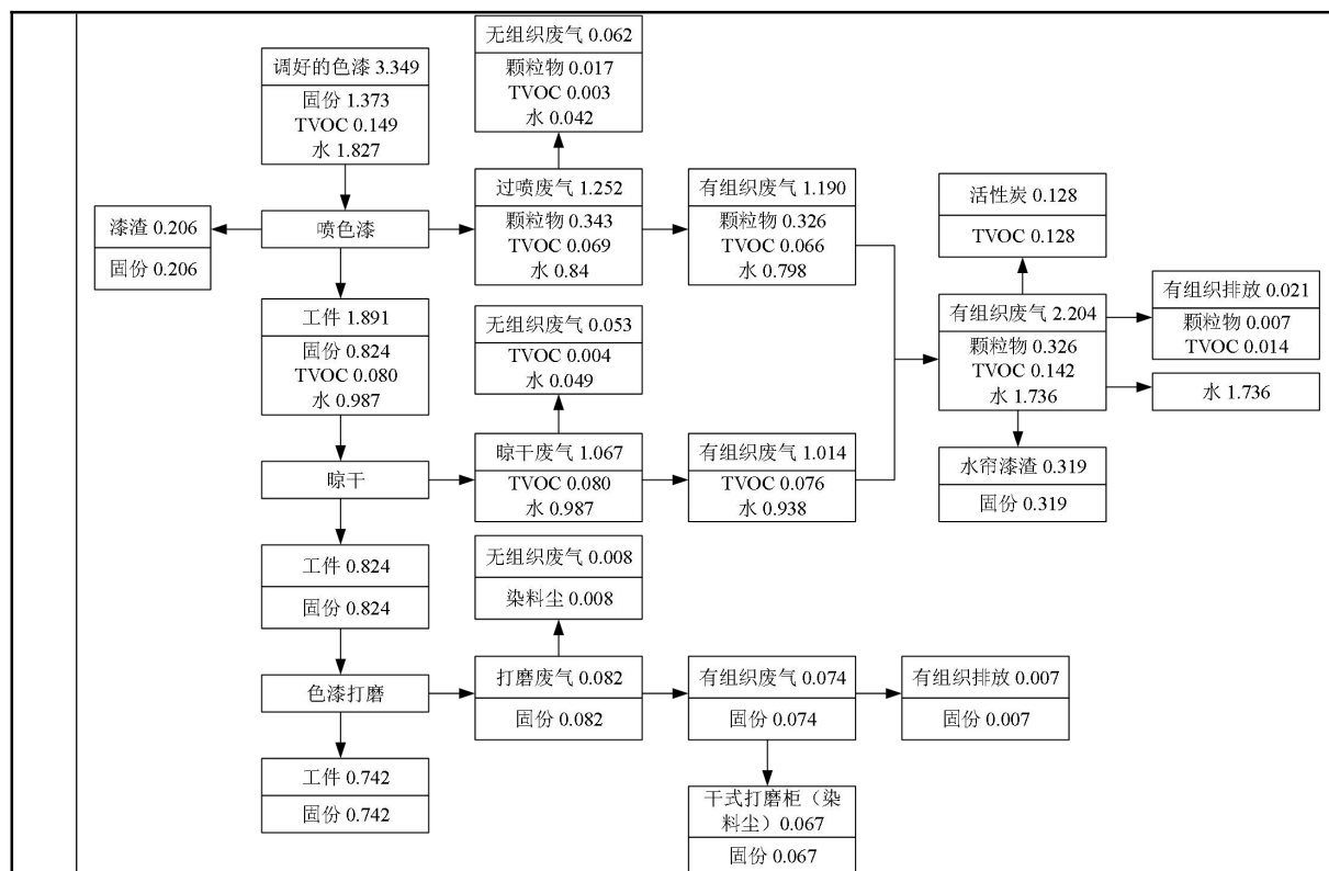
图 2-4 色漆物料平衡图 单位: t/a
