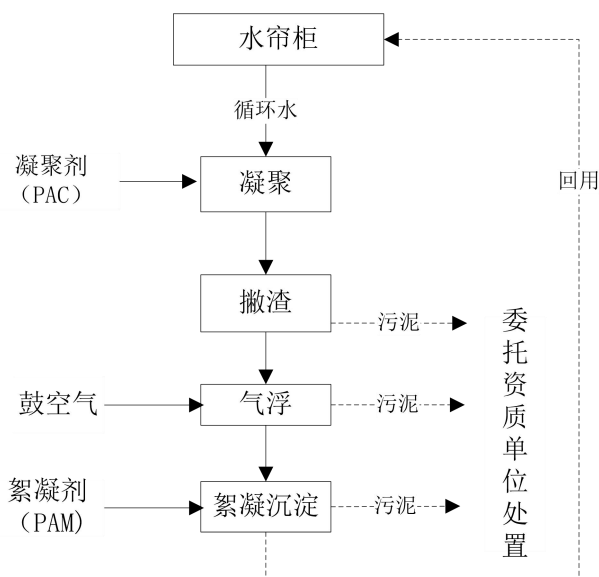
图 4-2 废水处理工艺流程图
