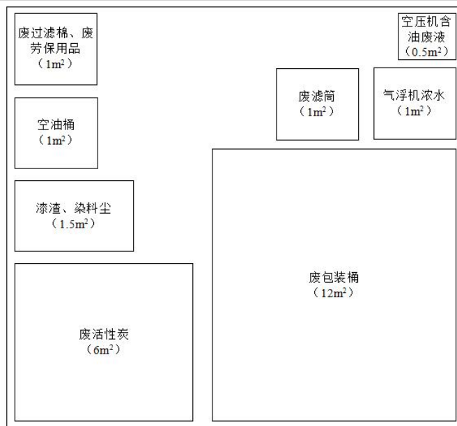
危废堆场分区存放图
