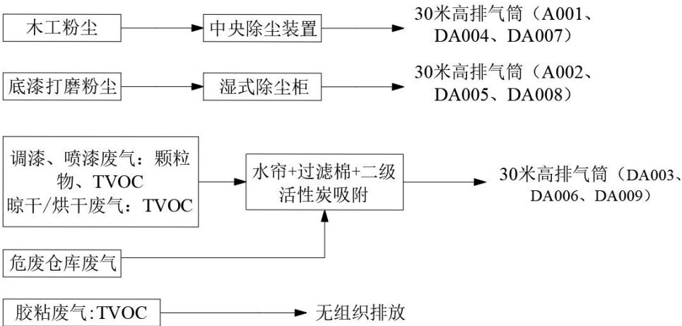
图 4-1 本项目废气收集、处理方式示意图
