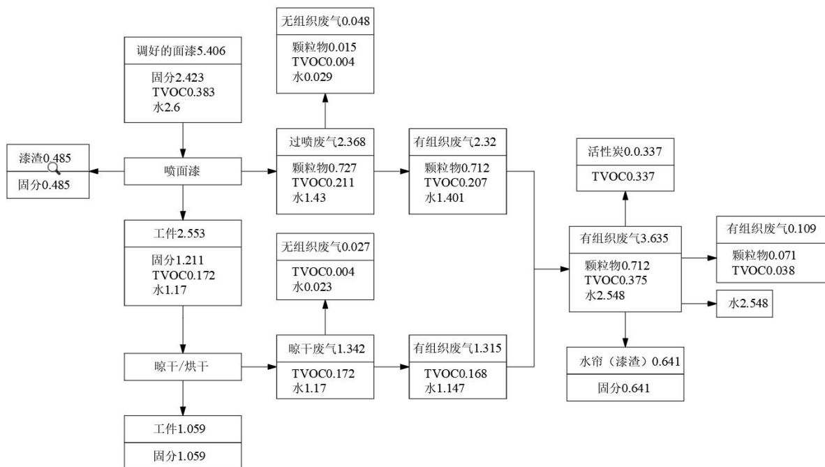
图 2-3 水性面漆物料衡图 单位: t/a
