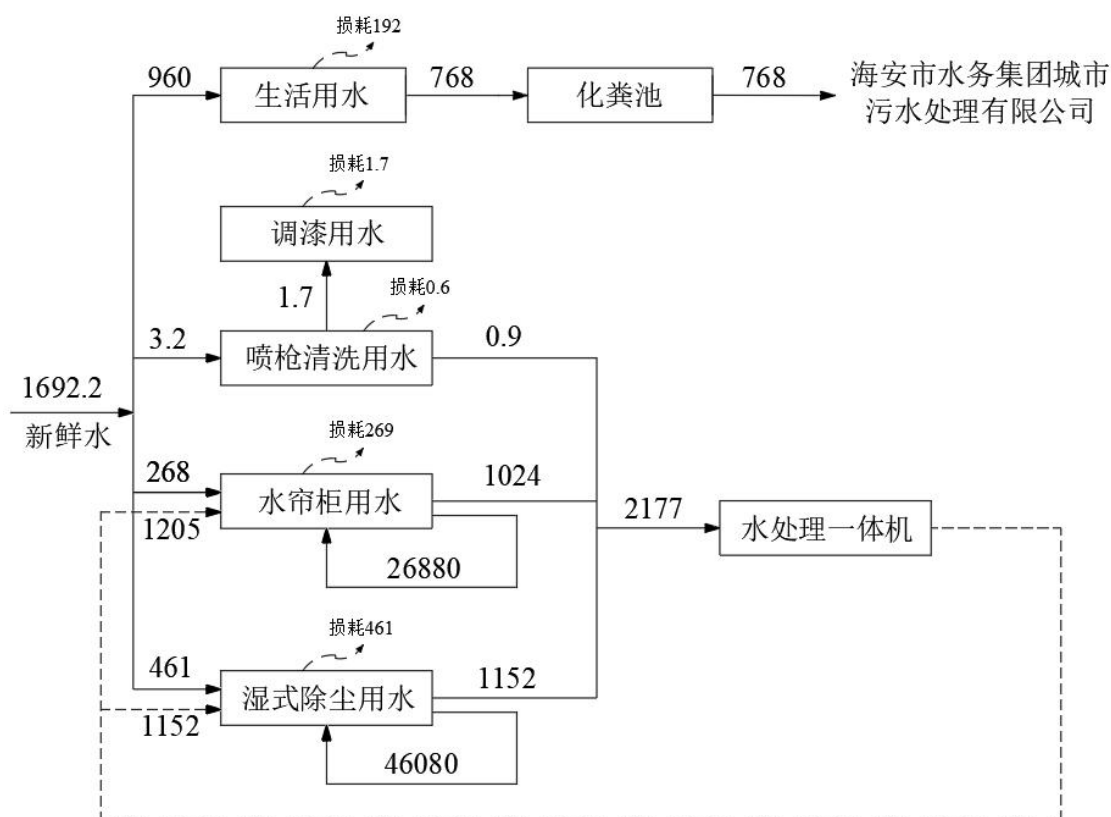
图 2-3 建设项目营运期水平衡图（单位：t/a）
