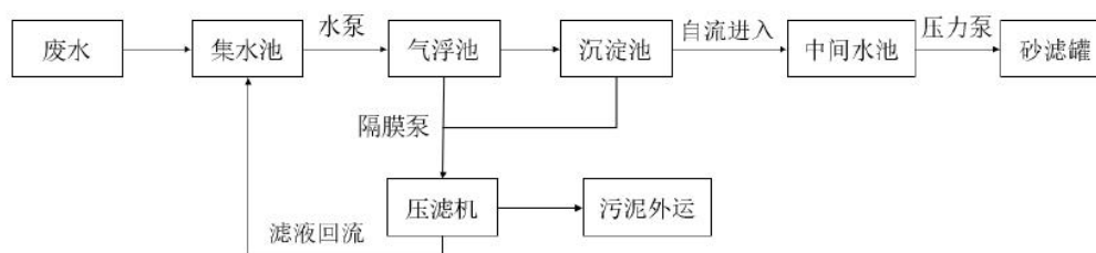
图 4-2 废水处理工艺流程示意图
