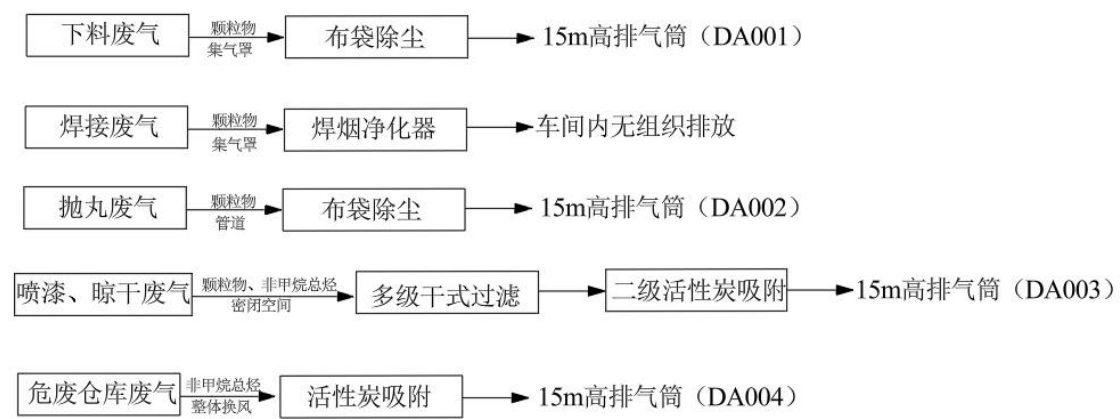
图 4-1 本项目废气收集、处理方式示意图
