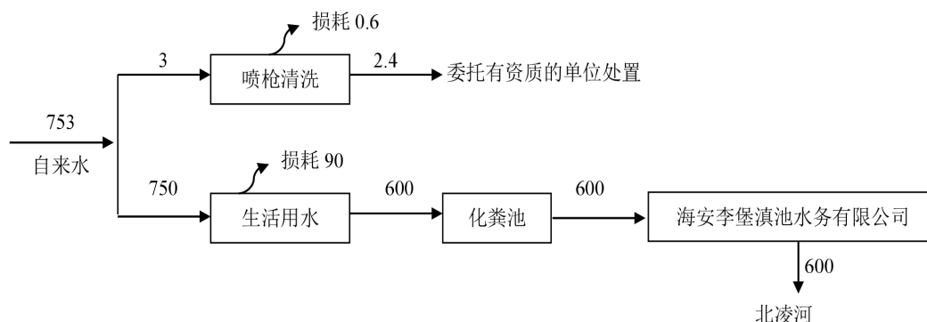
图 2-2 本项目营运期水平衡图（单位：t/a）
