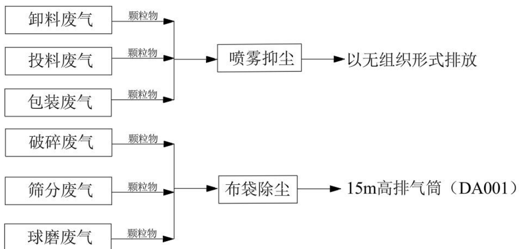
图 4-1 废气收集、处理方式示意图
