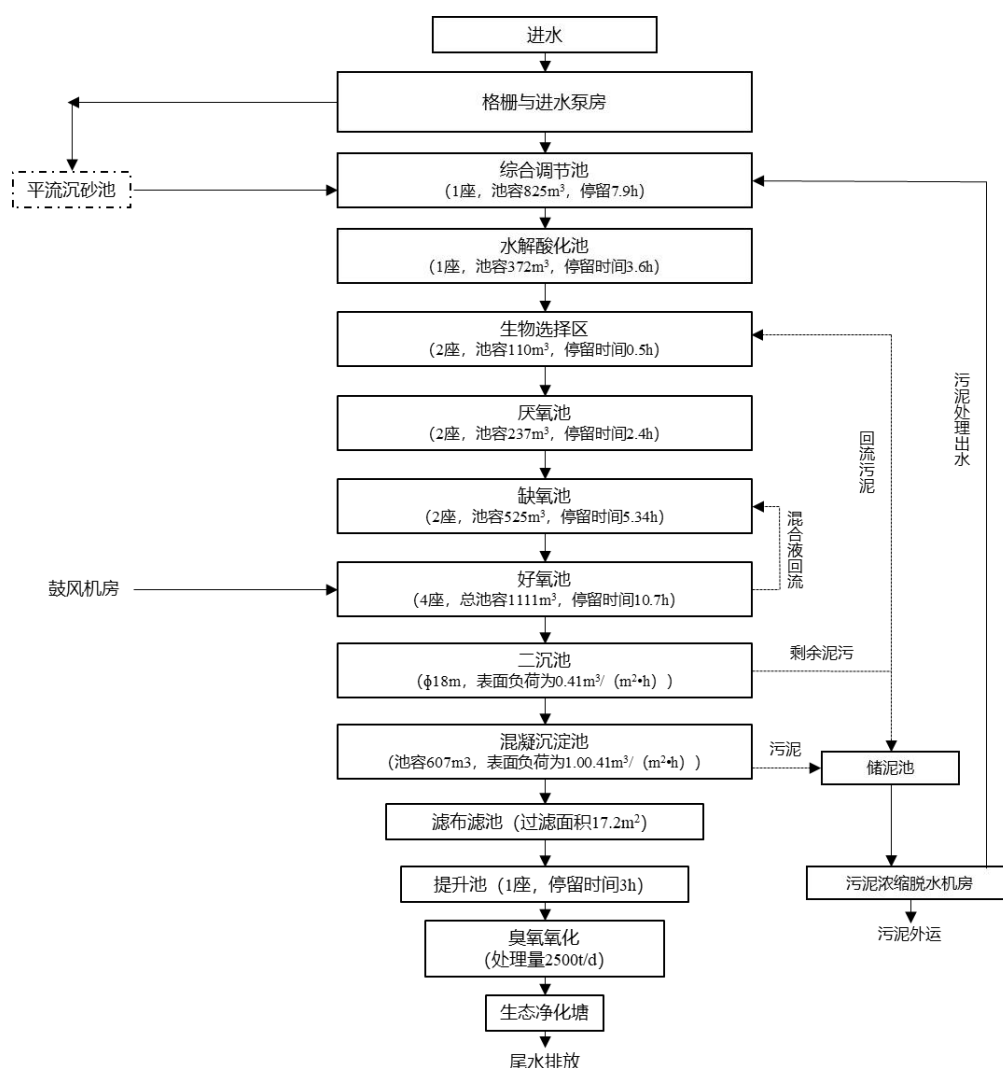
图 4-2 如皋市蒲涛污水处理有限公司处理工艺流程图
