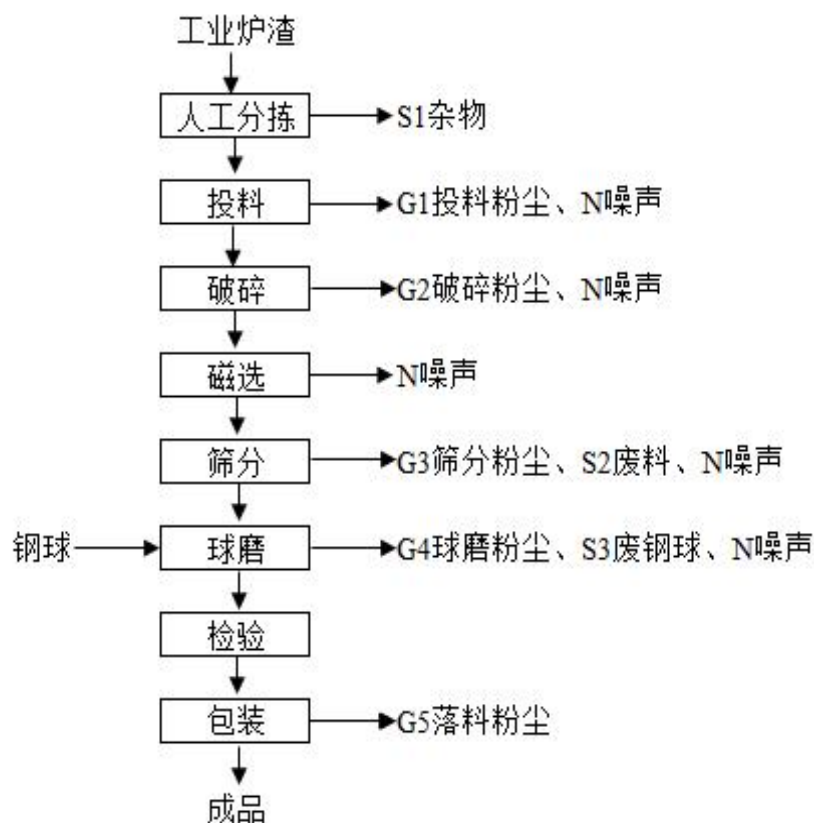
图 2-1 本项目工艺流程及产污节点示意图
