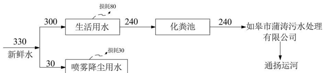
图 2-1 全厂水平衡图 (单位: t/a)
