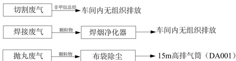
图 4-1 本项目废气收集、处理方式示意图
