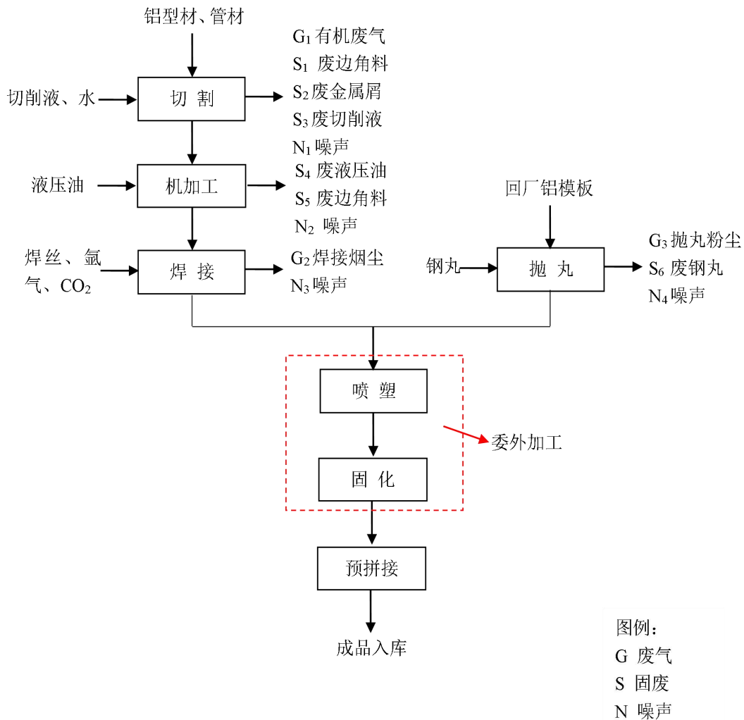
图 2-2 本项目生产工艺流程及产污节点示意图
