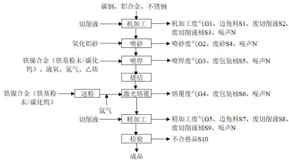
图 2-2 生产线工艺流程图
