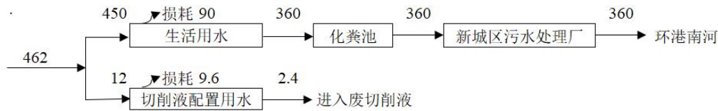
图 2-1 建设项目营运期水平衡图（单位：t/a）
