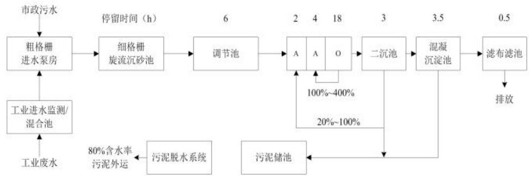
图 4-3 老坝港滨海新区污水处理厂工艺流程图
