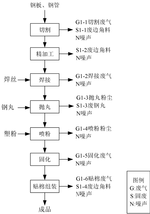
图2-3 金属餐桌椅生产工艺流程及产污节点图
