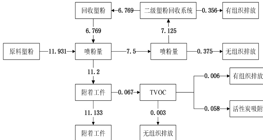
图 2-1 项目喷粉物料平衡图（单位：t/a）
