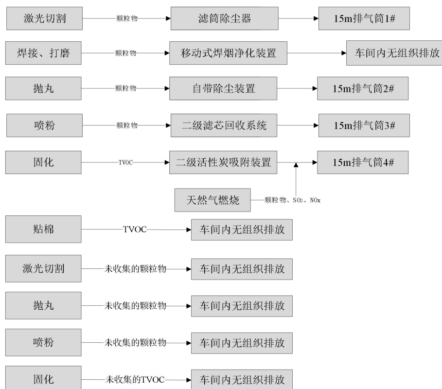
图 4-1 本项目废气收集、处理方式示意图
