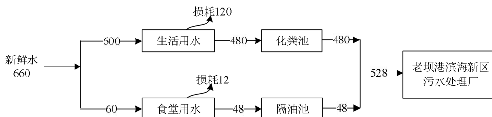
图 2-2 建设项目营运期水平衡图（单位：t/a）
