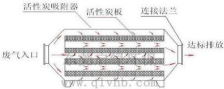
图 4-2 活性炭吸附原理图
