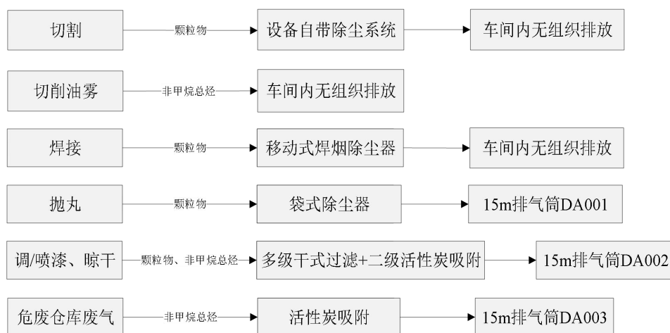
图 4-1 项目废气收集、处理方式示意图
