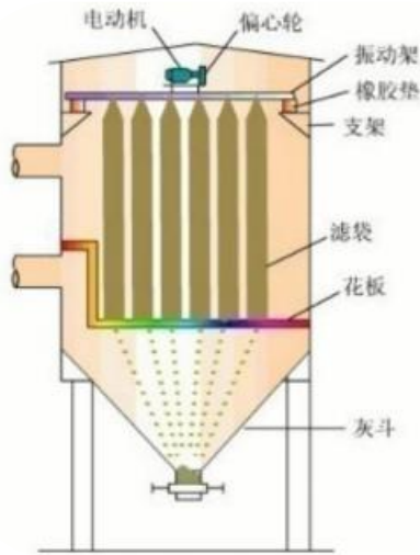
图 4-2 布袋除尘器结构示意图
