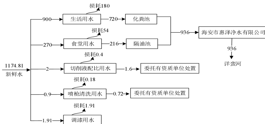
图 2-2 建设项目水平衡图 (单位: t/a)
