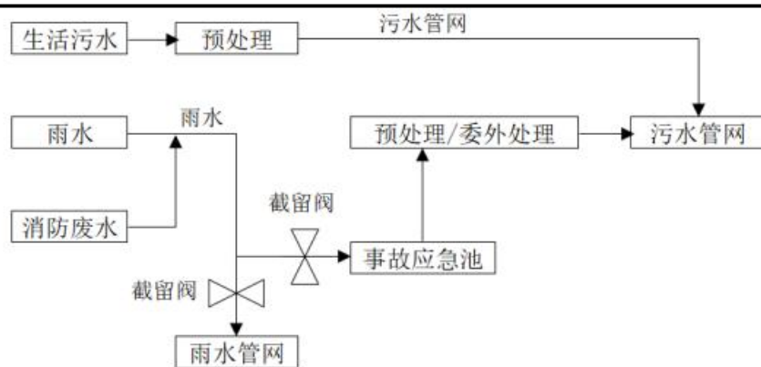
图 4-7 事故废水收集排放管网示意图
