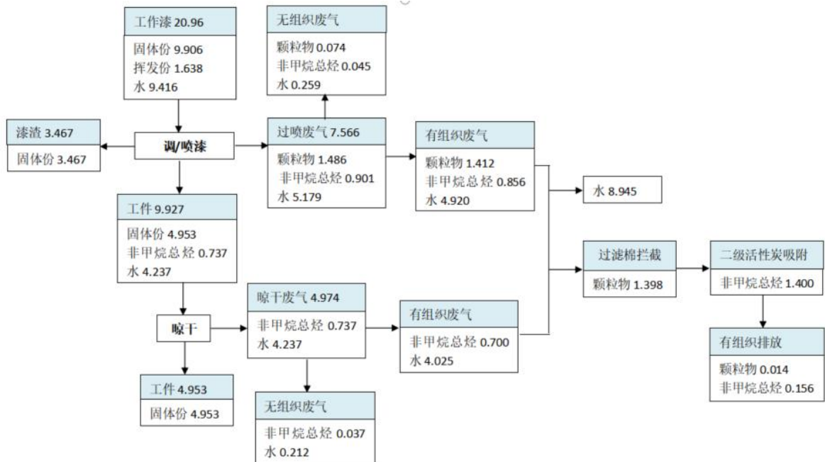
图 2-1 涂料物料平衡图 单位：t/a
