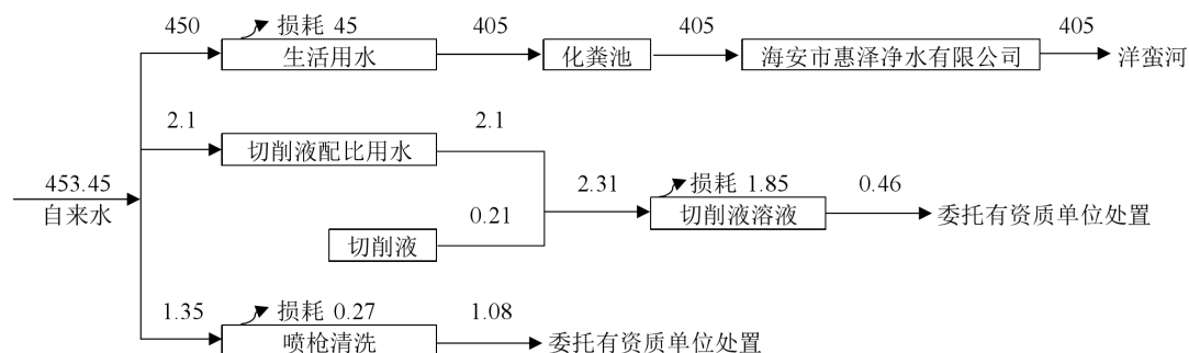
图 2-4 建设项目营运期水平衡图 (单位: t/a)
