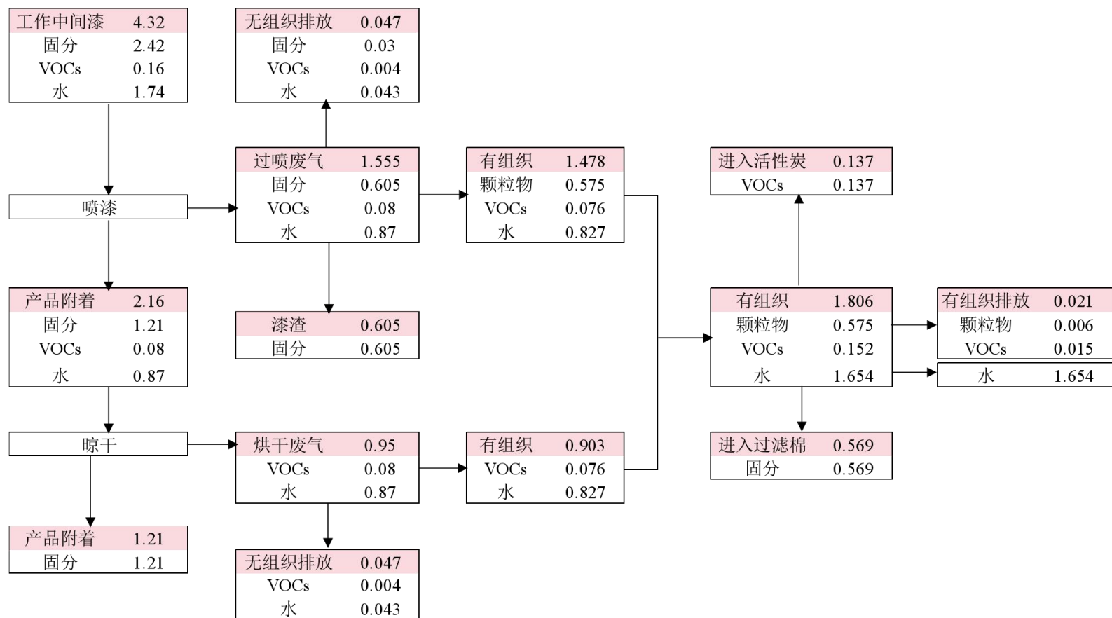
图 2-2 工作中间漆物料平衡图（单位：t/a）
