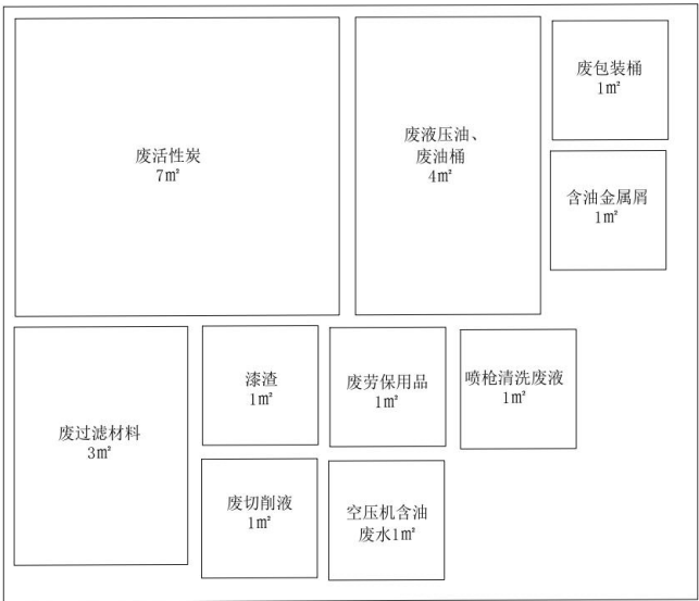
图 4-4 危废仓库布置图
