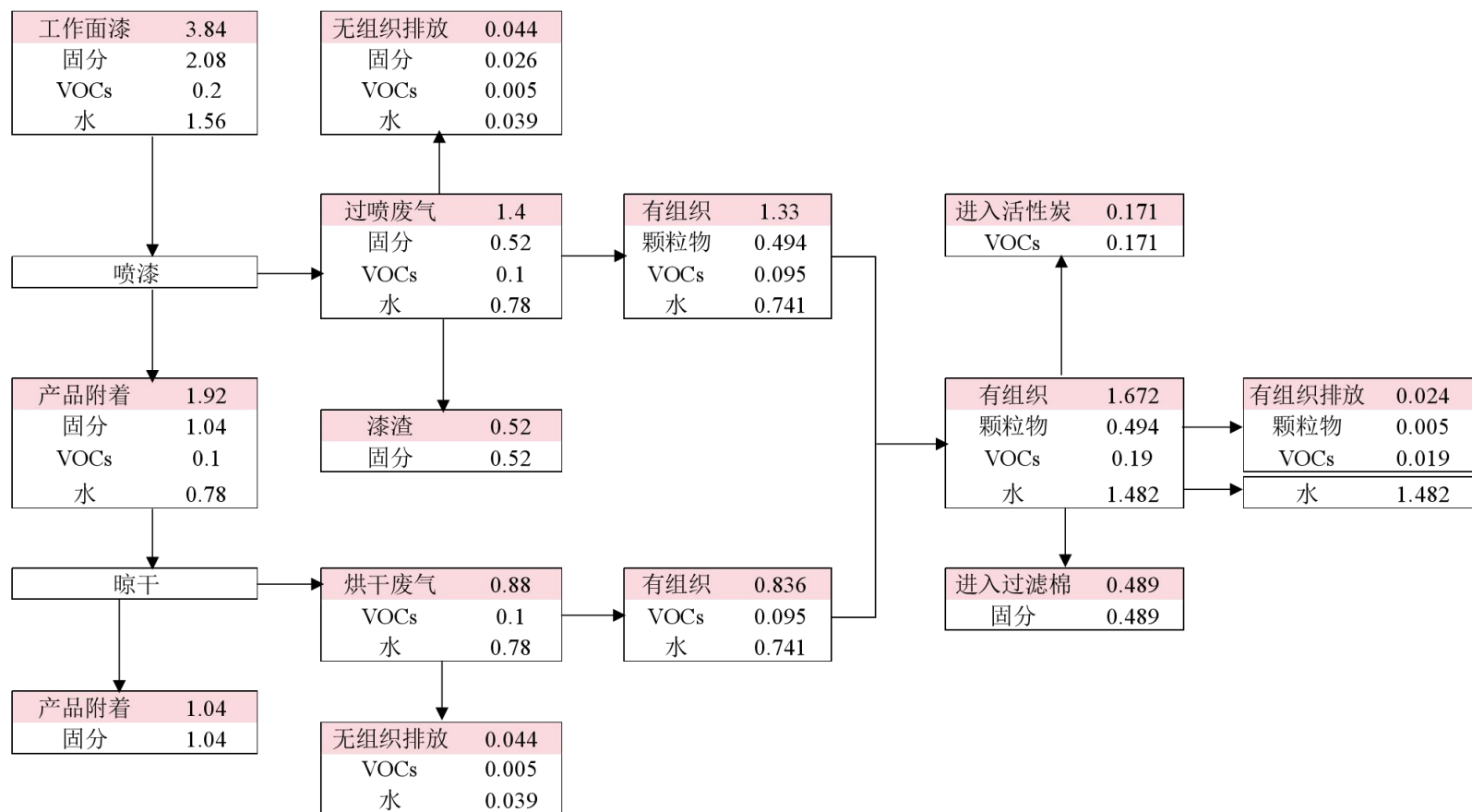
图 2-3 工作面漆物料平衡图（单位：t/a）
