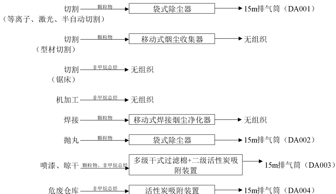
图 4-1 废气处置方式示意图
