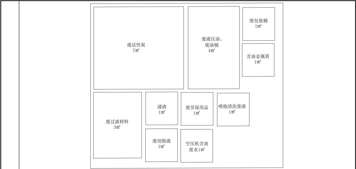
图 4-4 危废仓库布置图
