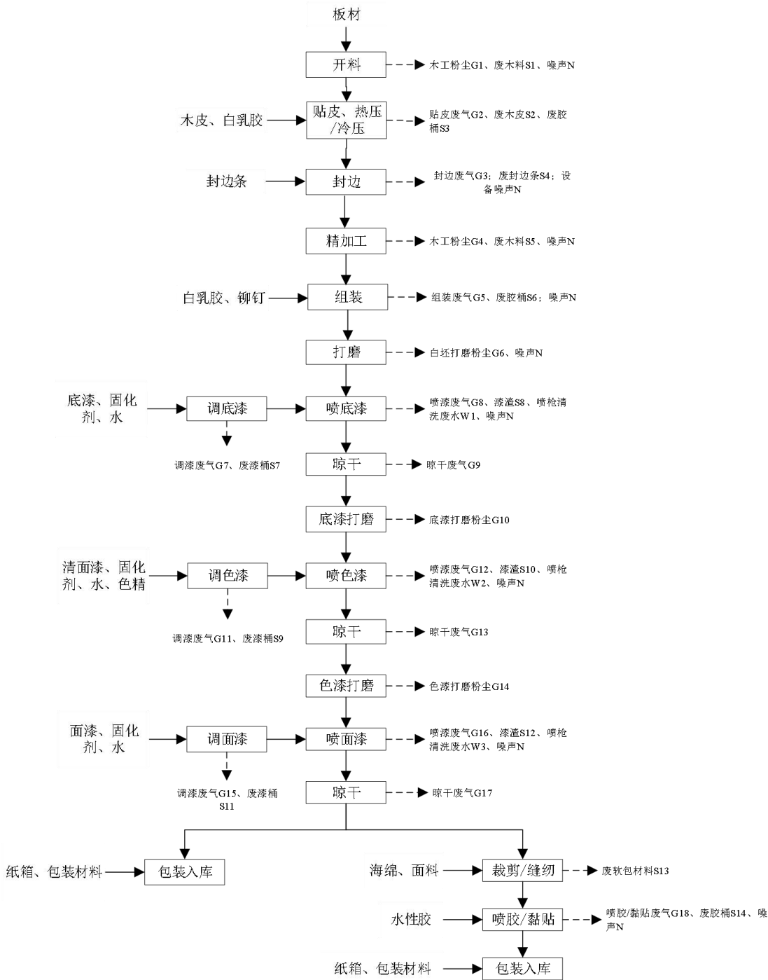
图 2-7 酒店家具工艺流程及产污环节图
