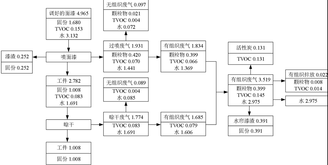
图 2-3 面漆物料平衡图 单位：t/a
