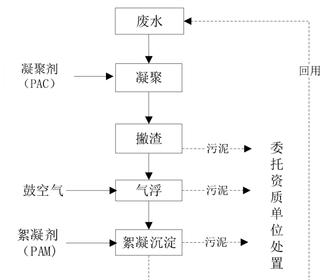
图 4-1 废水处理工艺流程图
