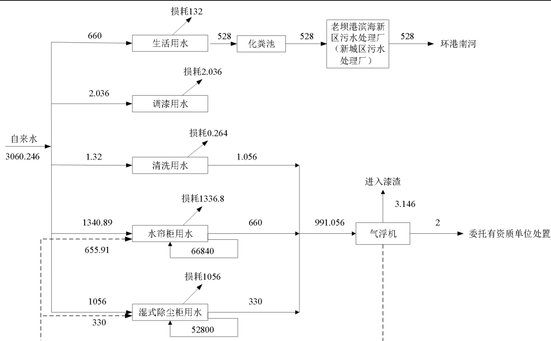
图 2-6 建设项目营运期水平衡图 (单位: t/a)
