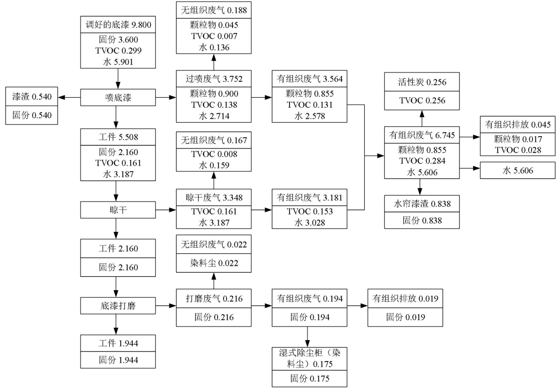
图 2-2 底漆物料平衡图 单位：t/a
