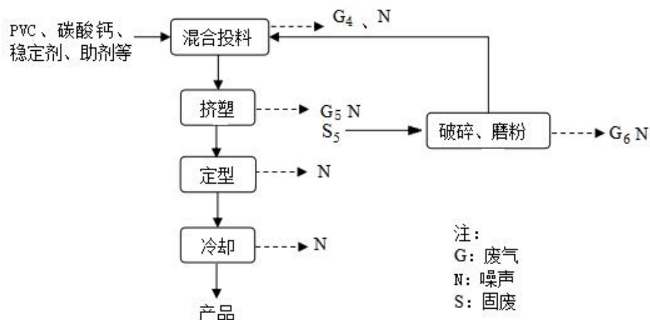
图 2-3 管材生产工艺流程图
