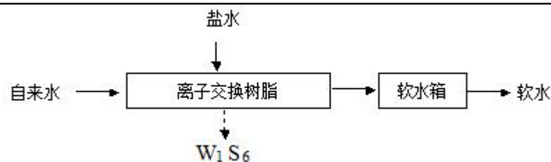
图 2-4 软水制备工艺流程图
