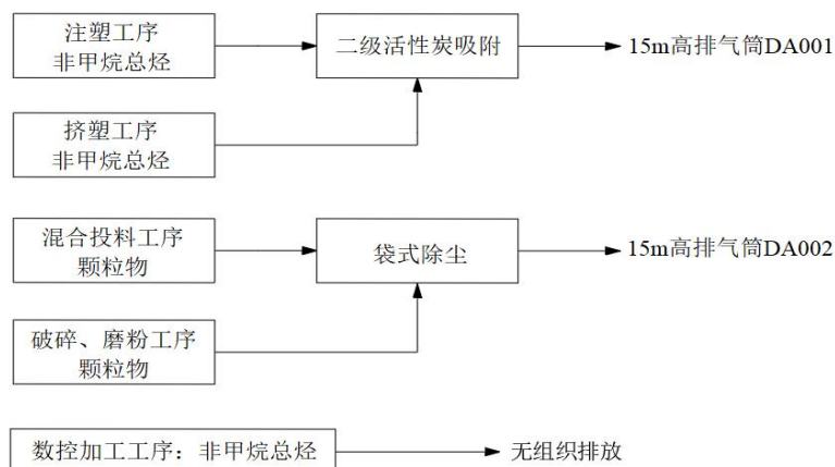
图 4-1 项目废气处理及排放方式图
