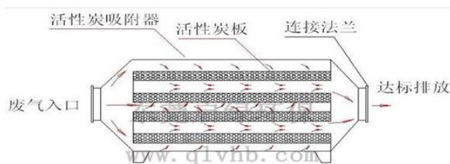
图 4-2 项目活性炭吸附器装置示意图
