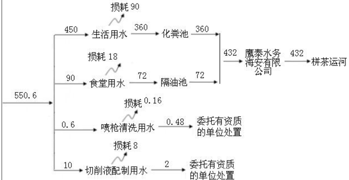
图 2-2 建设项目营运期水平衡图 (单位: t/a)
