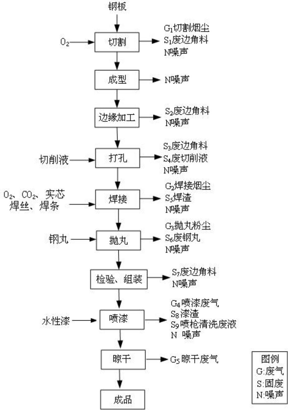
图2-3 生产工艺流程及产污节点图
