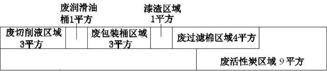
图 4-4 危废仓库布置图
