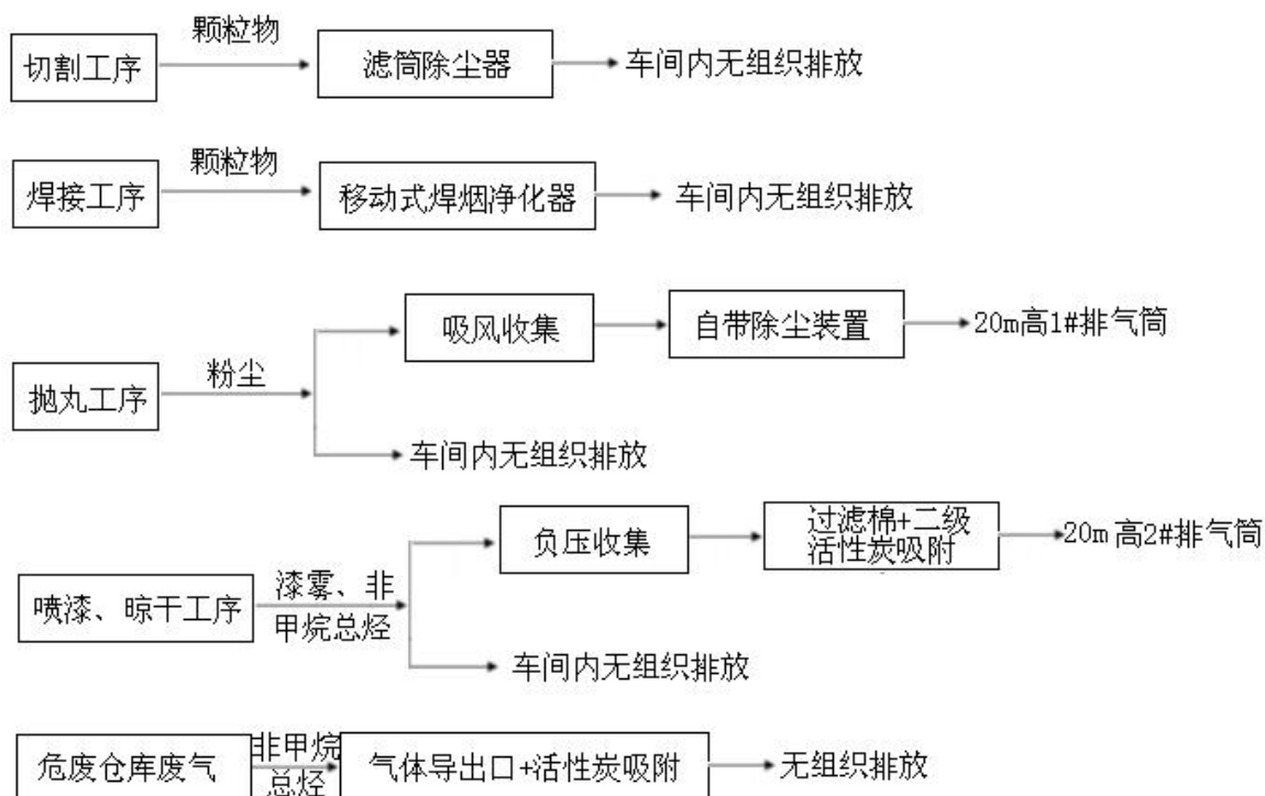
图 4-1 本项目废气收集、处理方式示意图
