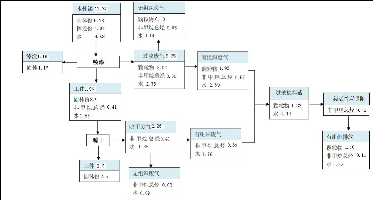
图 2-1 水性漆物料衡图 单位: t/a
