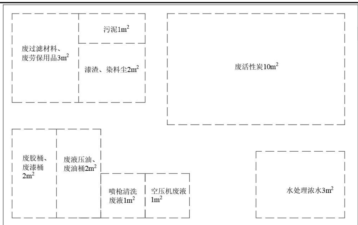
图 4-5 危废仓库布置图
