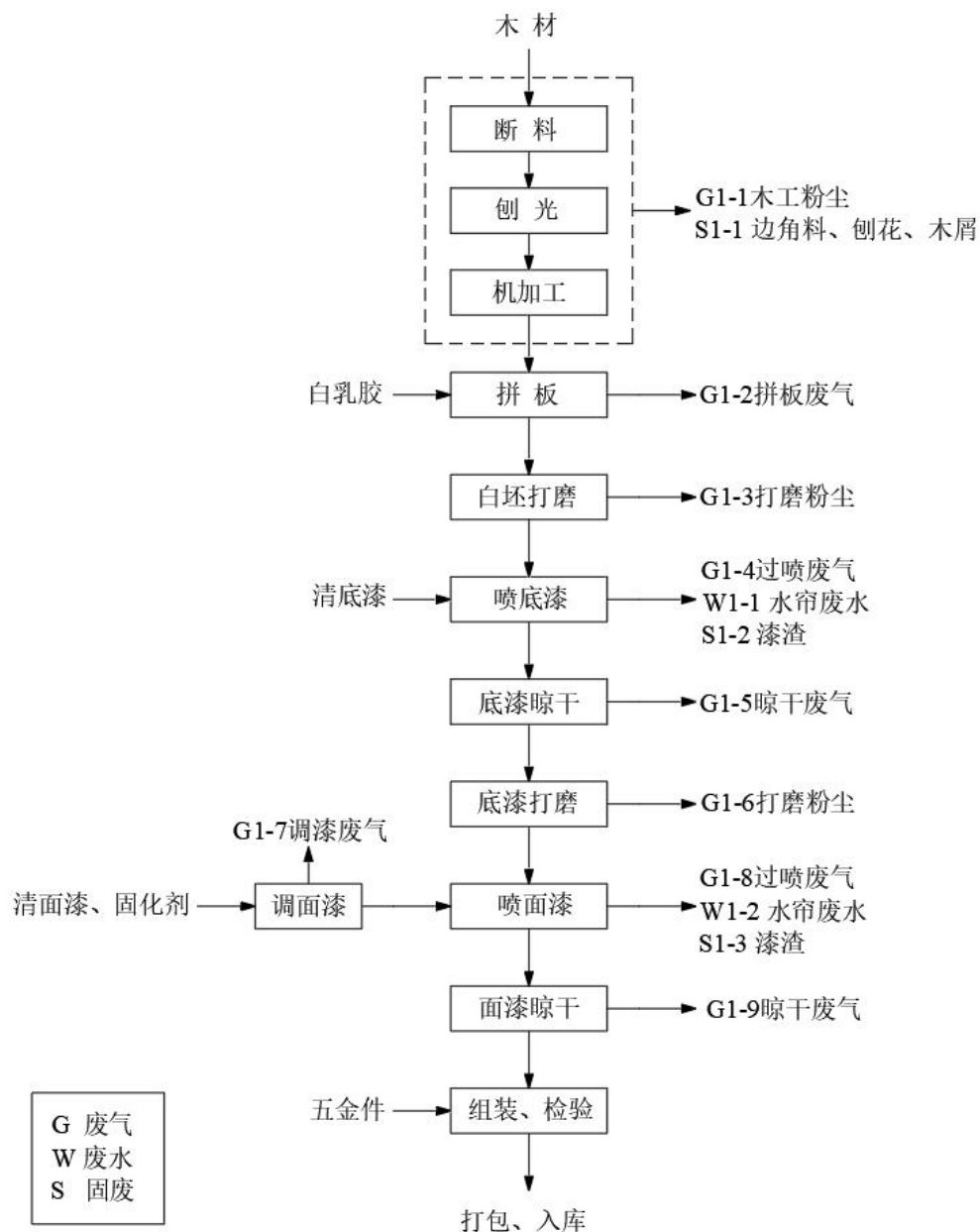
图 2-3 实木家具生产工艺流程及产污节点示意图
