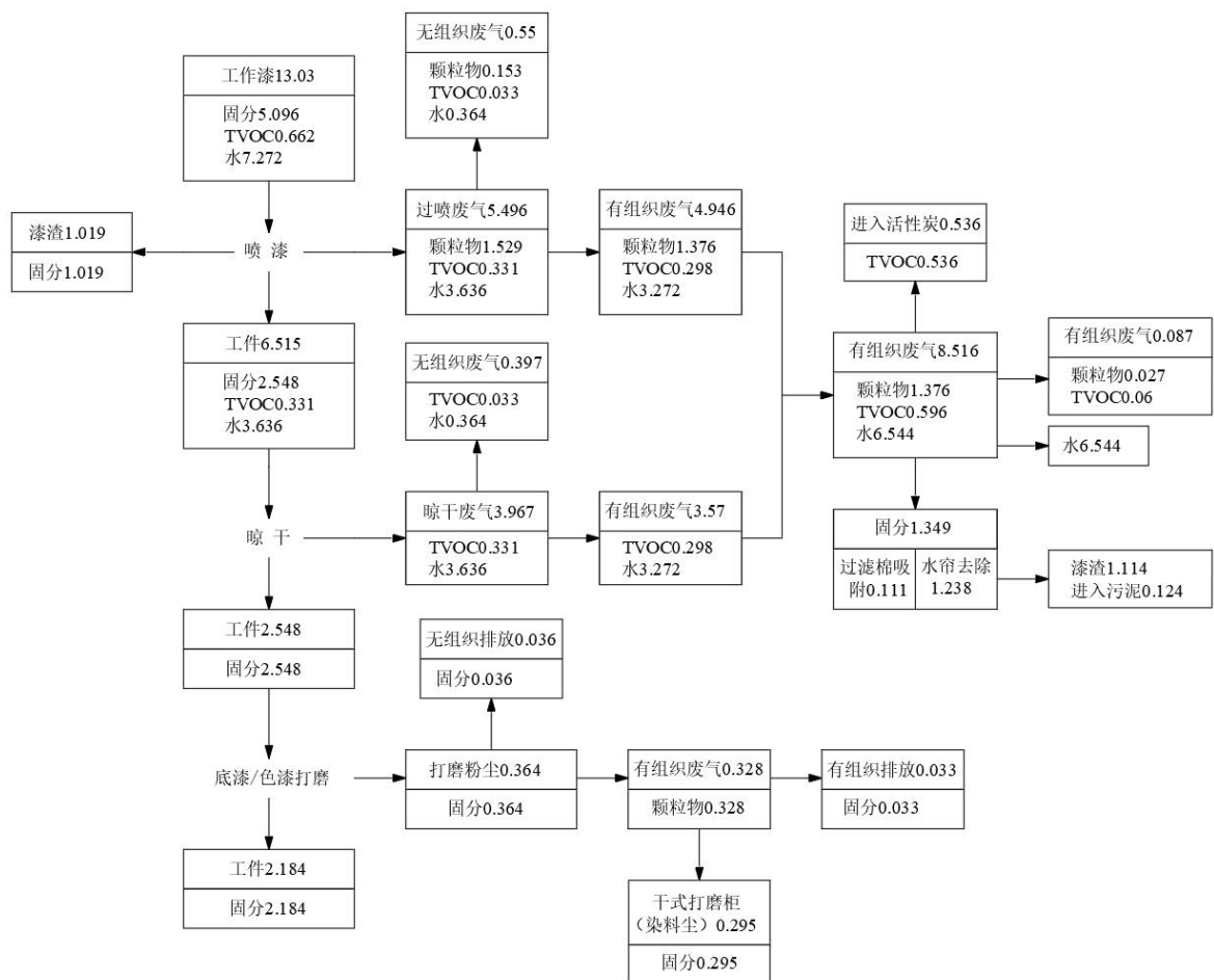
图 2-1 水性漆物料平衡图 单位：t/a
