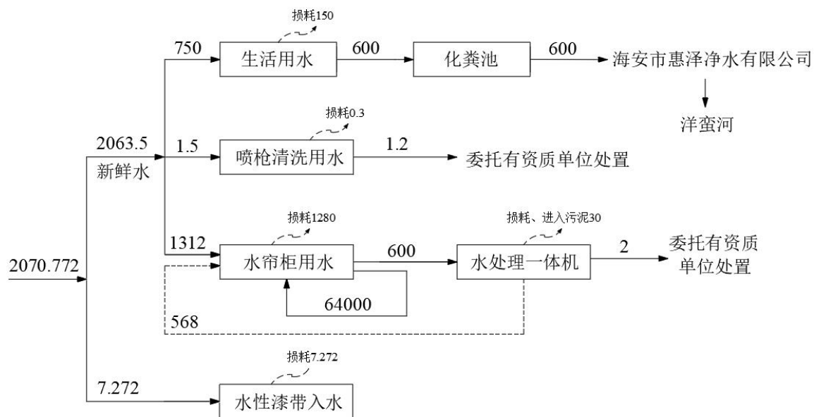
图 2-2 营运期水平衡图 (单位: t/a)
