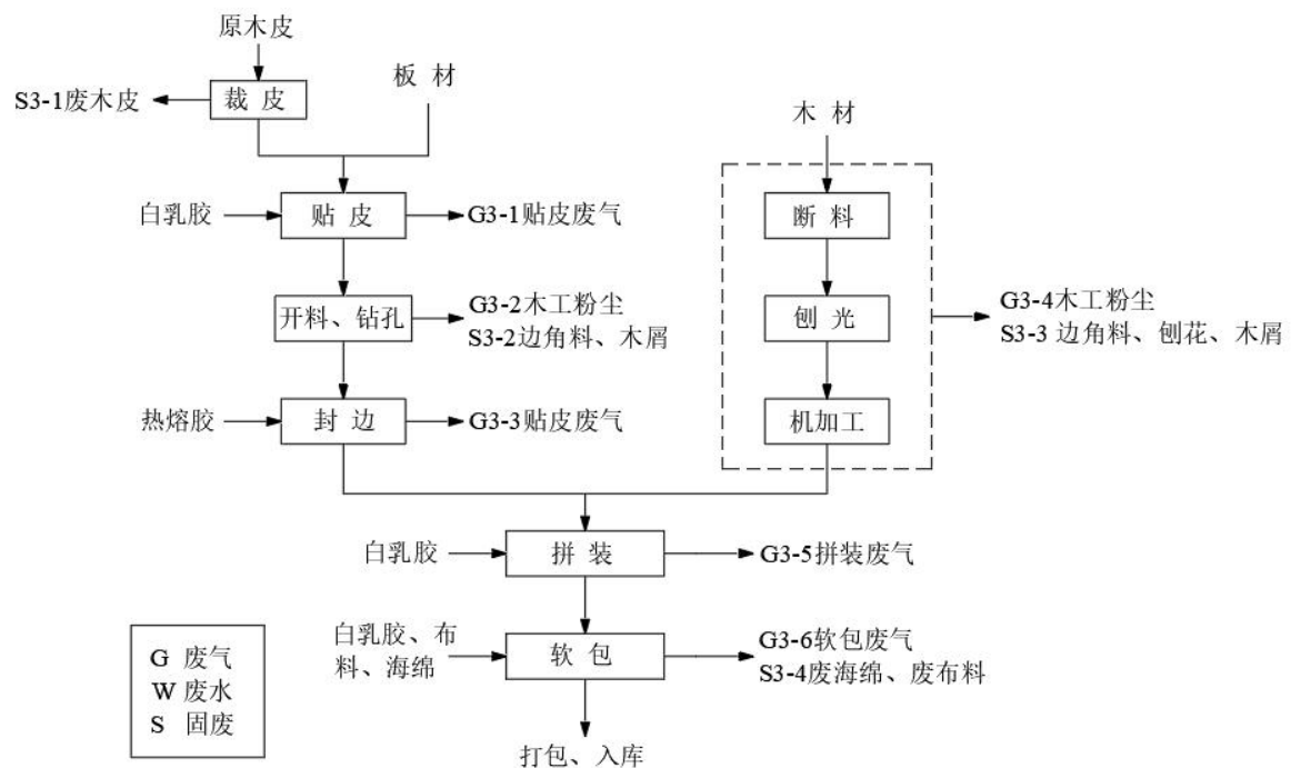
图 2-5 软包家具生产工艺流程及产污节点示意图
