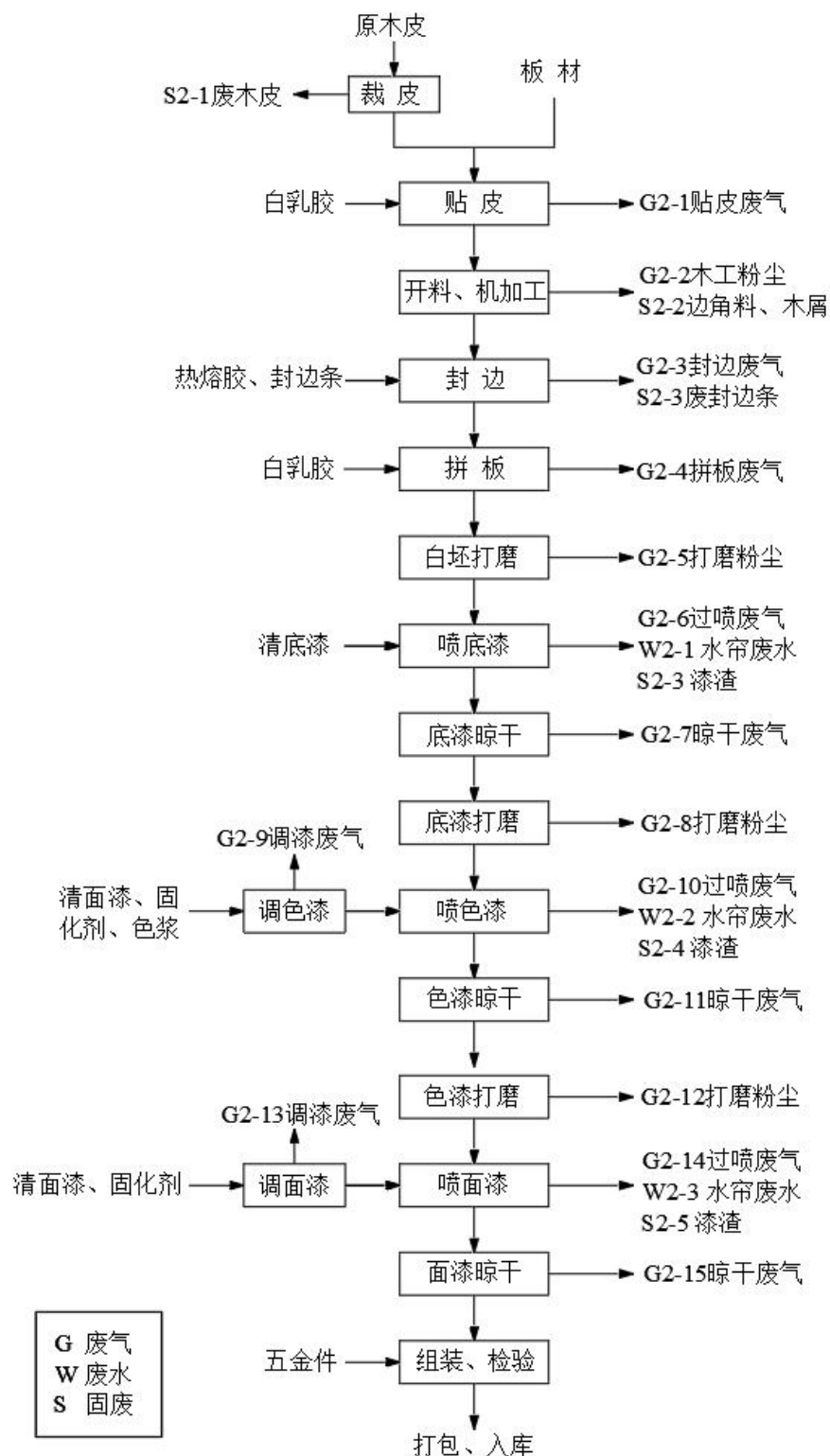
图 2-4 板式家具生产工艺流程及产污节点示意图
