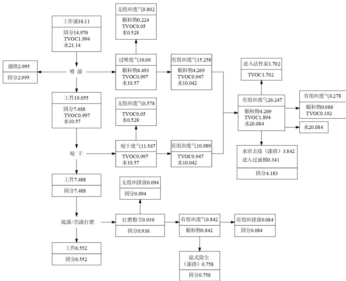
图 2-1 水性木器漆物料衡图 单位：t/a
