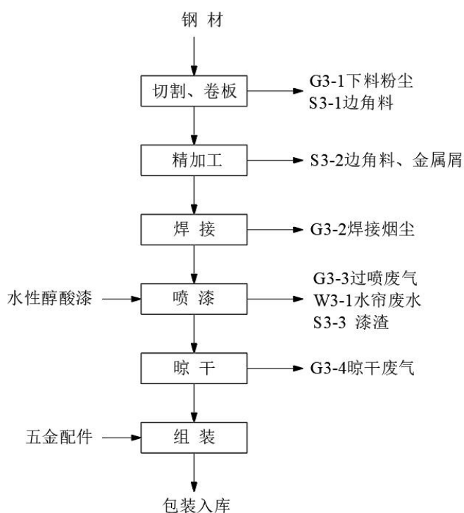
图 2-5 金属家具生产工艺流程及产污节点示意图
