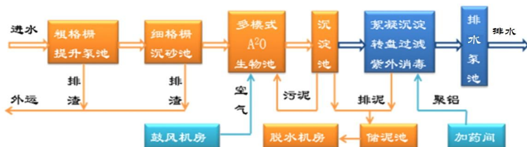
图 4-3 新城区污水处理厂处理工艺流程图
