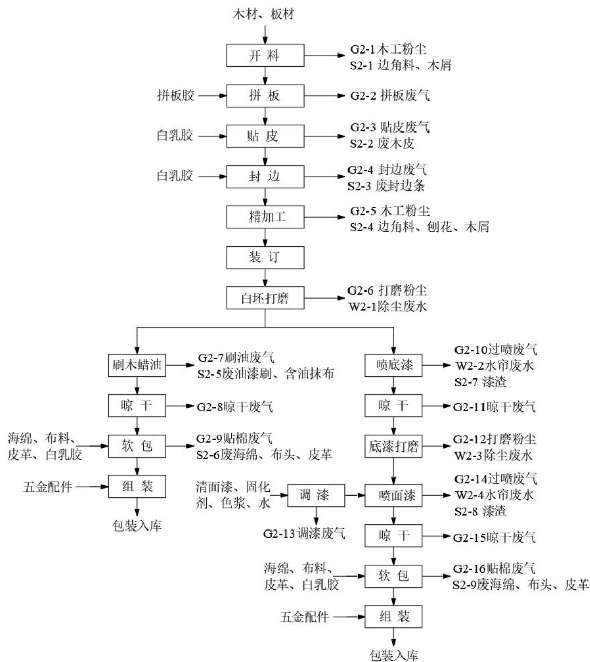
图 2-4 喷涂类木质家具生产工艺流程及产污节点示意图
