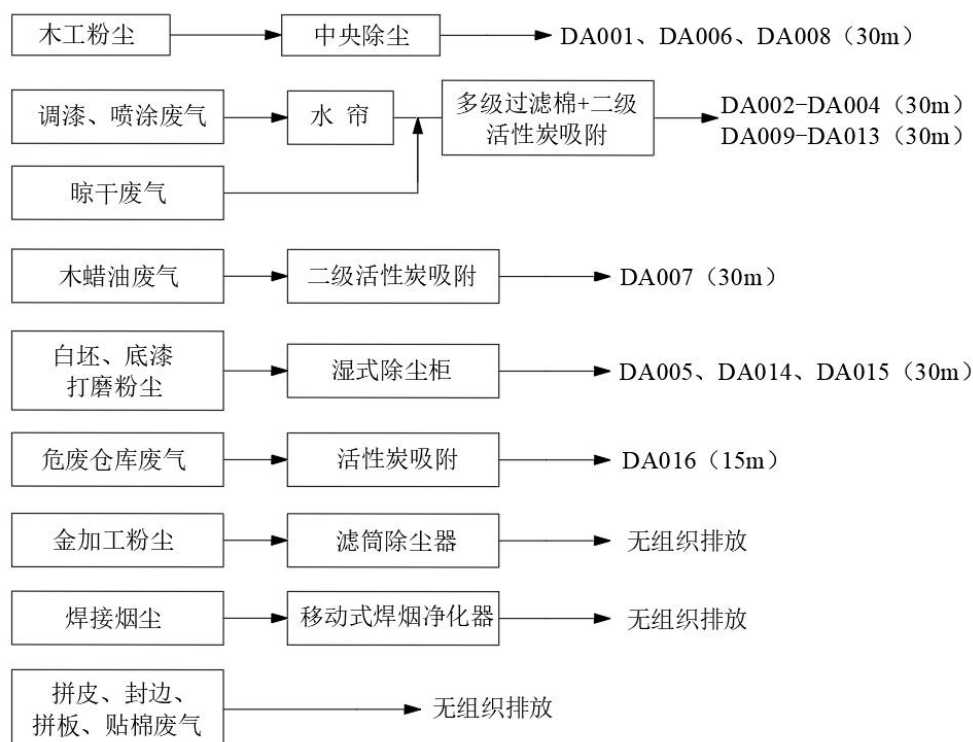
图 4-1 本项目废气收集、处理方式示意图
