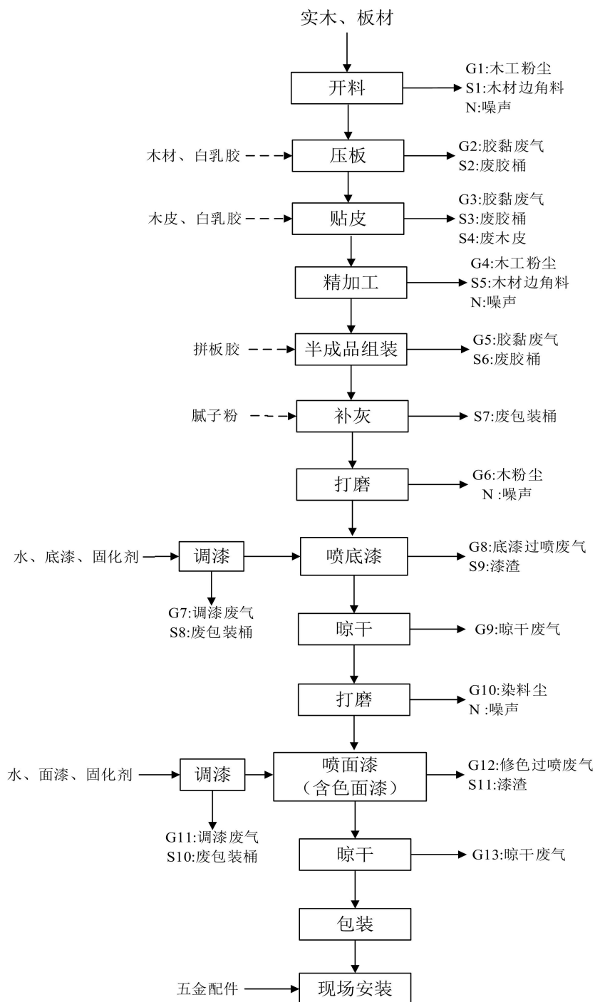
图 2-4 现有项目生产工艺及产排污节点示意图
