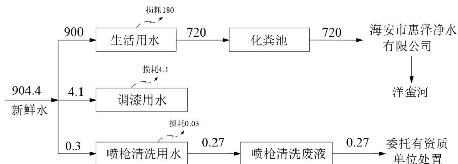
图 2-2 扩建项目营运期水平衡图（单位：t/a）
