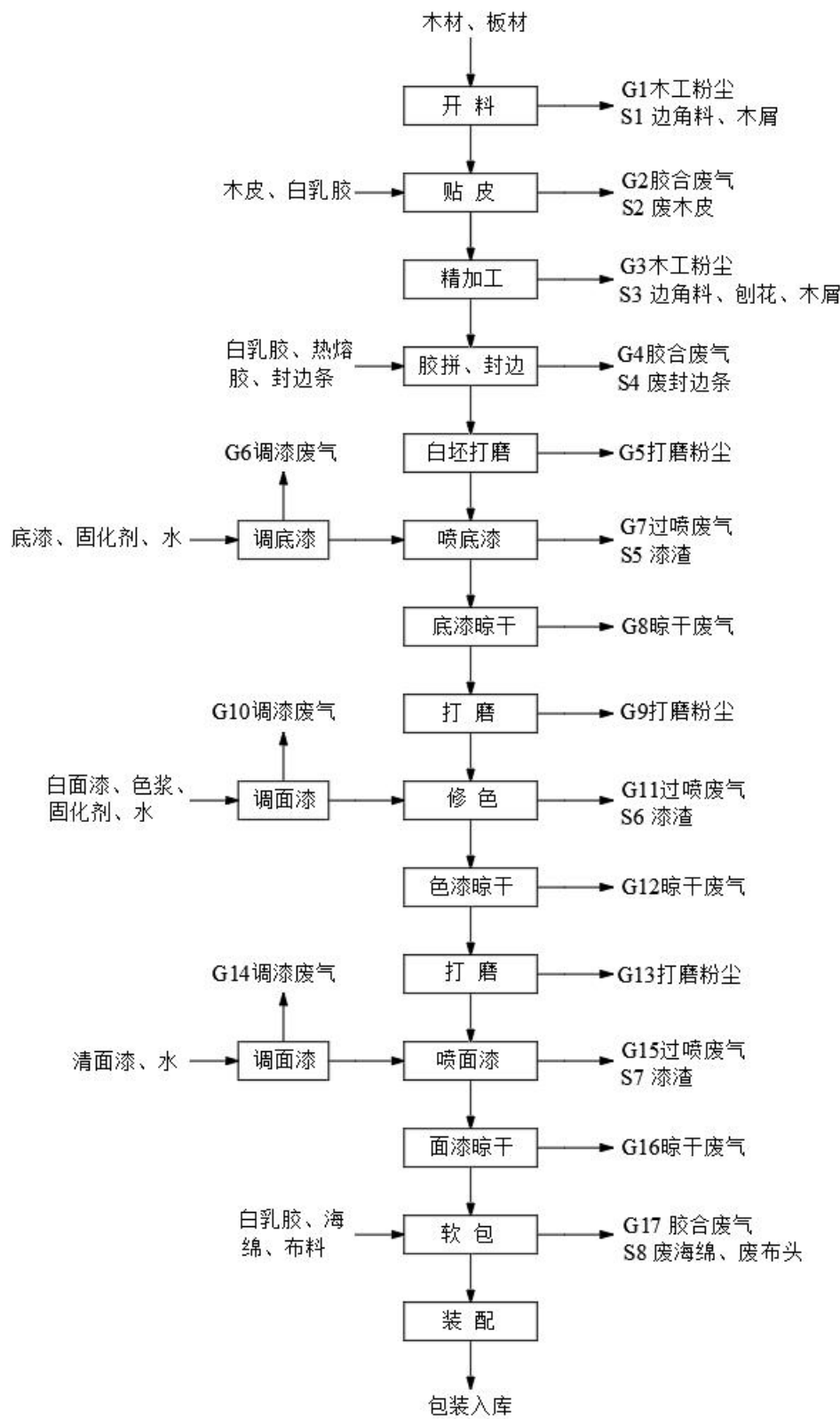
图 2-3 扩建项目生产工艺流程及产污节点示意图
