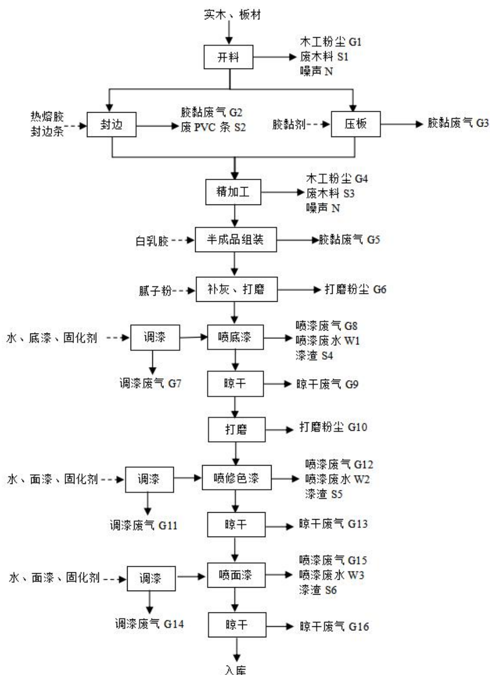
图 2-4 现有项目生产工艺及产排污节点示意图
