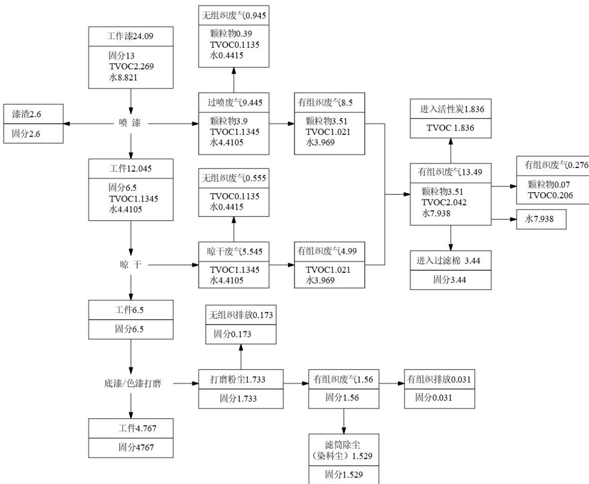
图 2-1 涂料物料衡图 单位：t/a
