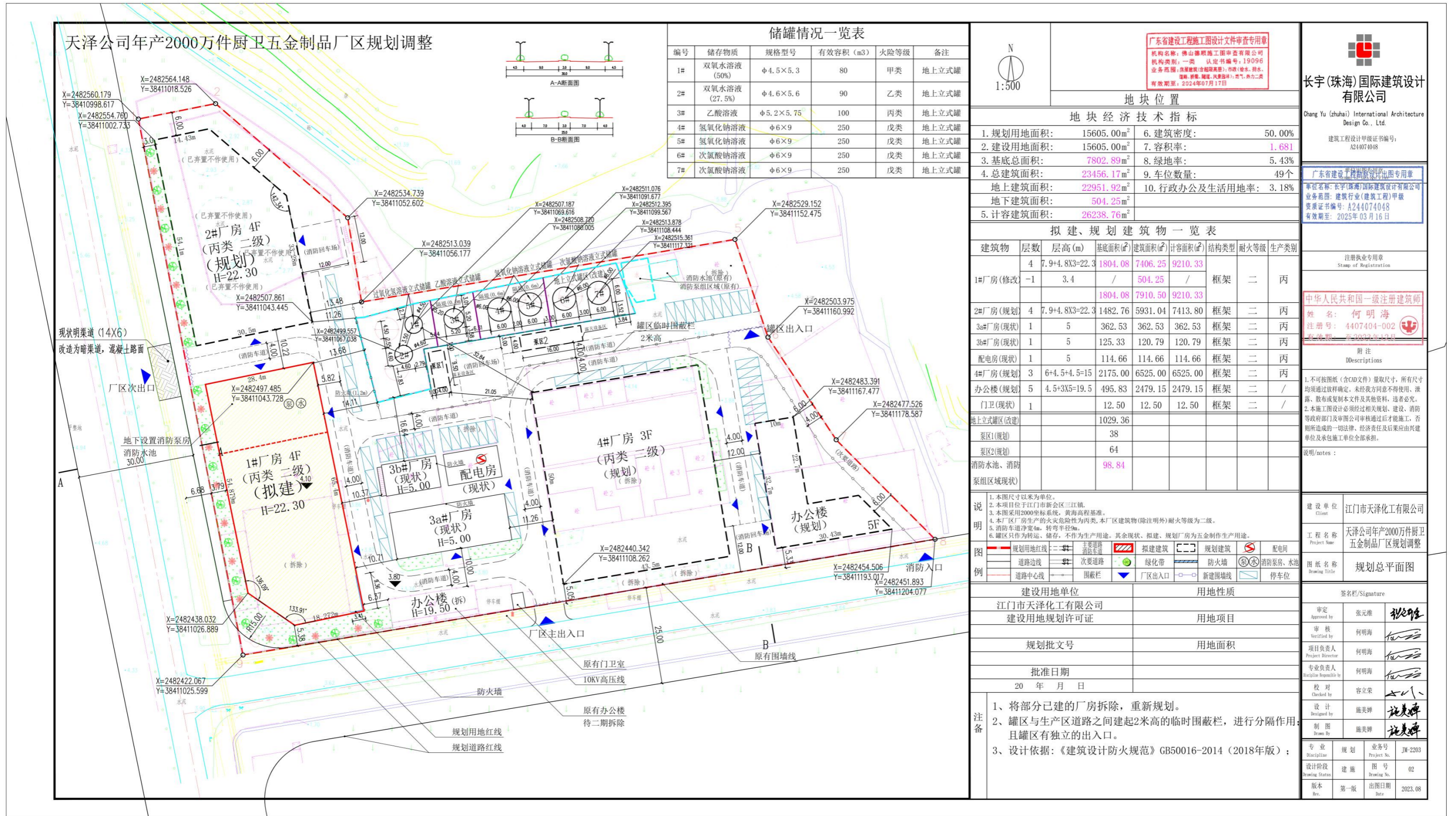
附图6：项目总体布置图
