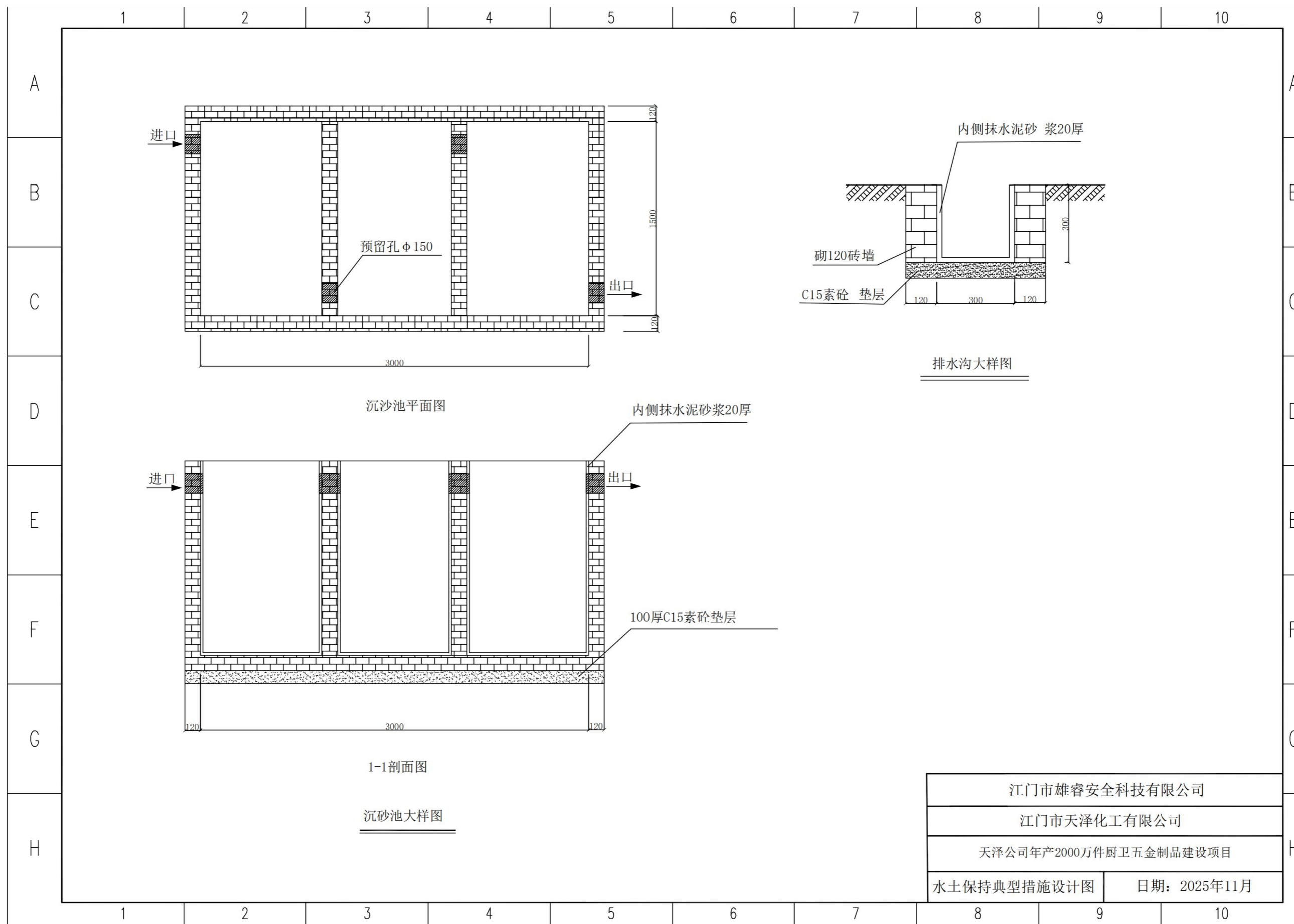
附图 8：水土保持典型措施设计图
