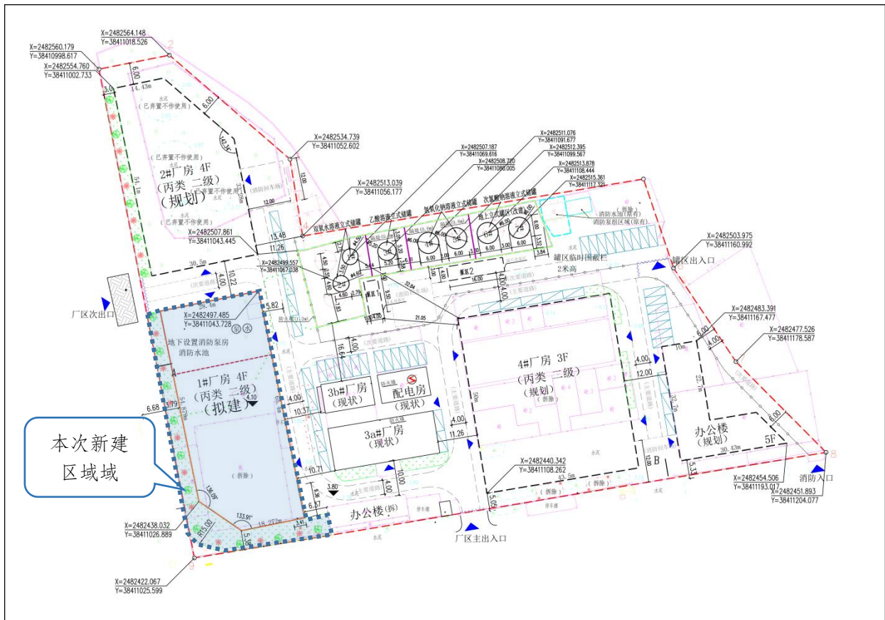
图 1-1 厂房布置图
