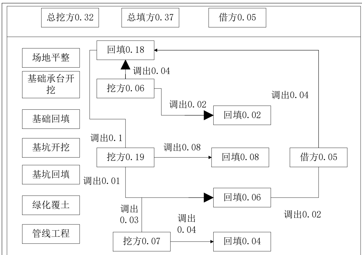
图 1-1 土石方流向框图 (万 m 3 )
