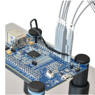
对于信号针脚位置在一起并没有足够的接地针脚的接头。可使用接地导线来连接测试中设备上的远程接地针脚。
