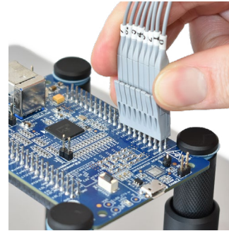
对于信号针脚在一排上而接地针脚在另一排上的接头。
