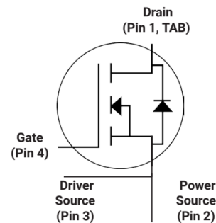
TO-247-4 Package
