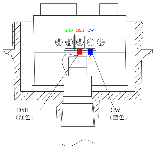
图 3.5 整体接线图
