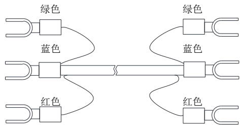
图 6.4 分体线外形图
