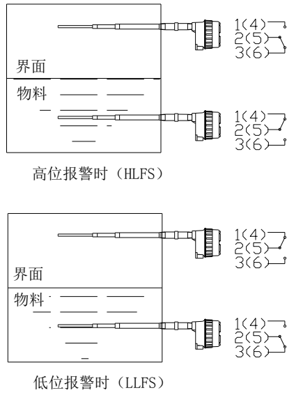
图 3.8 正常工作时继电器触点位置示意图
