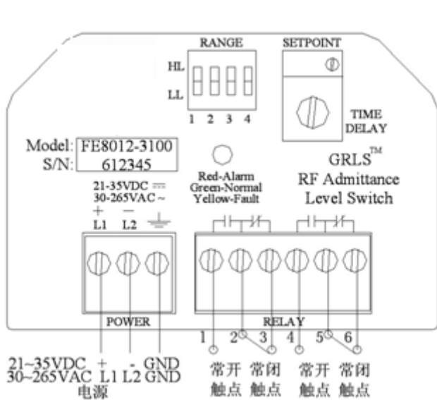
图 3.7 电源及继电器触点图
