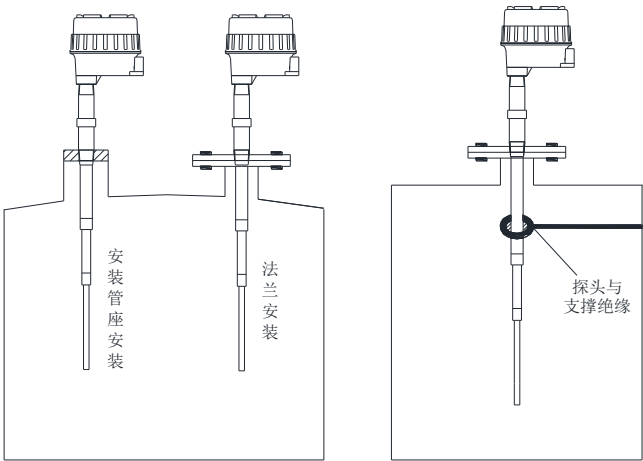
安装管座安装和法兰安装 固定支撑安装
