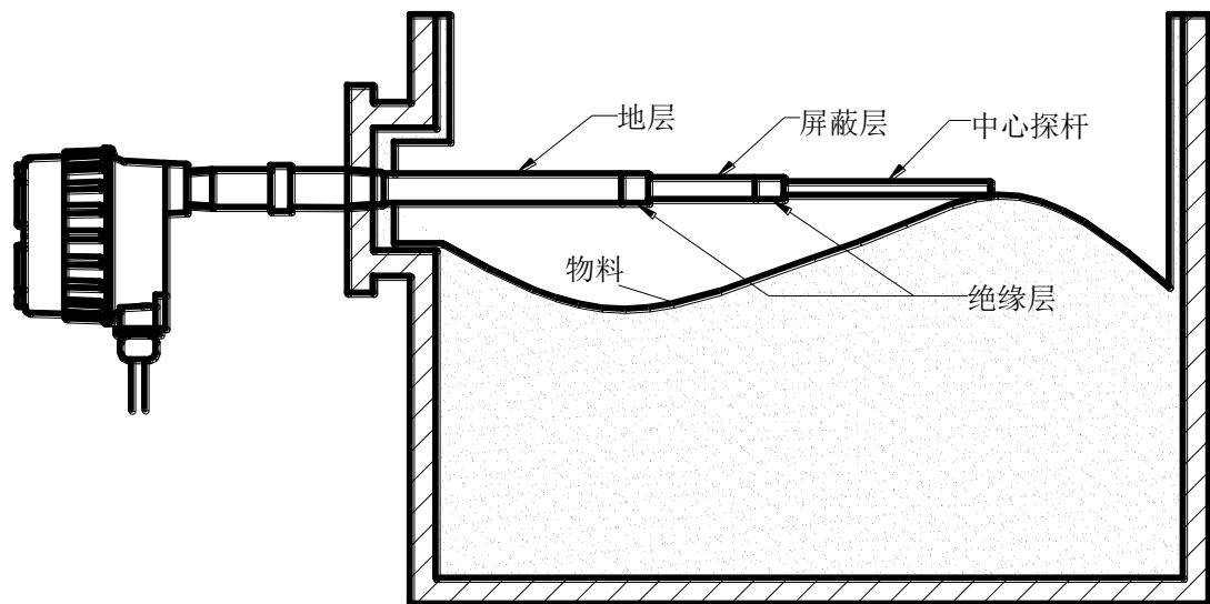
图 1.2 传感器结构
