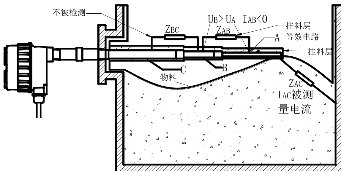
图 1.3 测量的等效示意图
