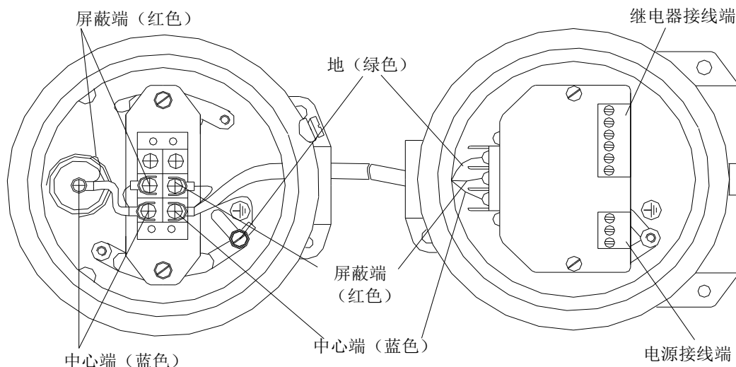
图 3.6 分体接线图
