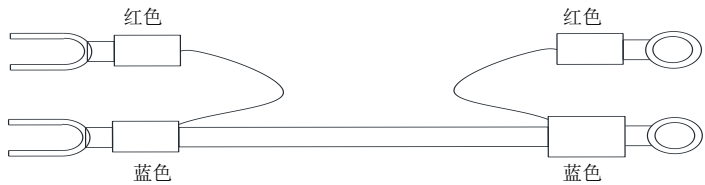
图 6.3 整体线外形图
