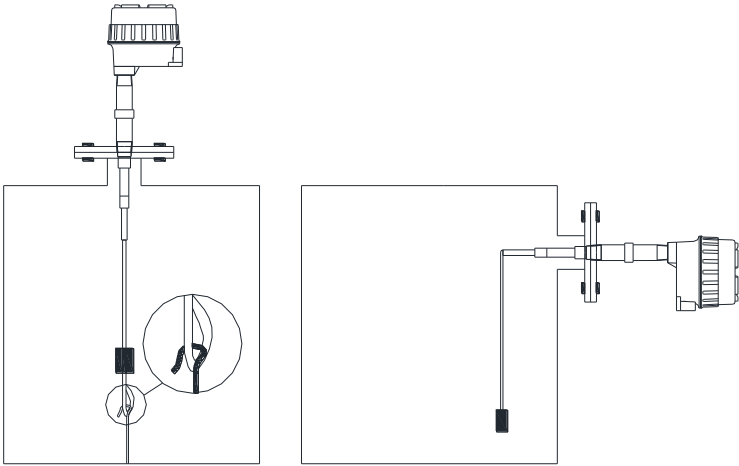
地锚安装 钓鱼杆式安装
