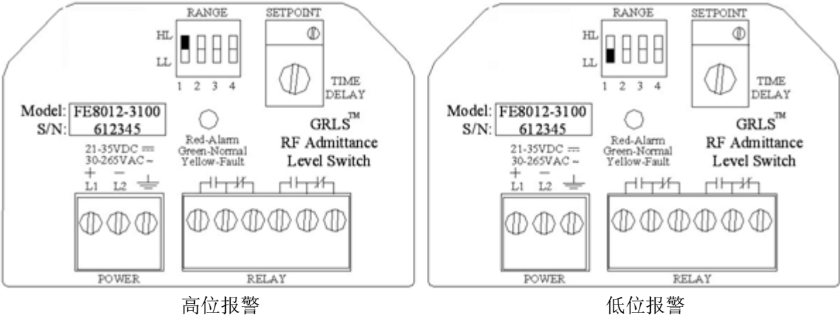
图 4.1 高低位报警方式
