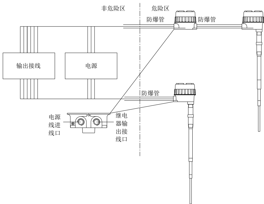
图 3.4 系统接线示意图
