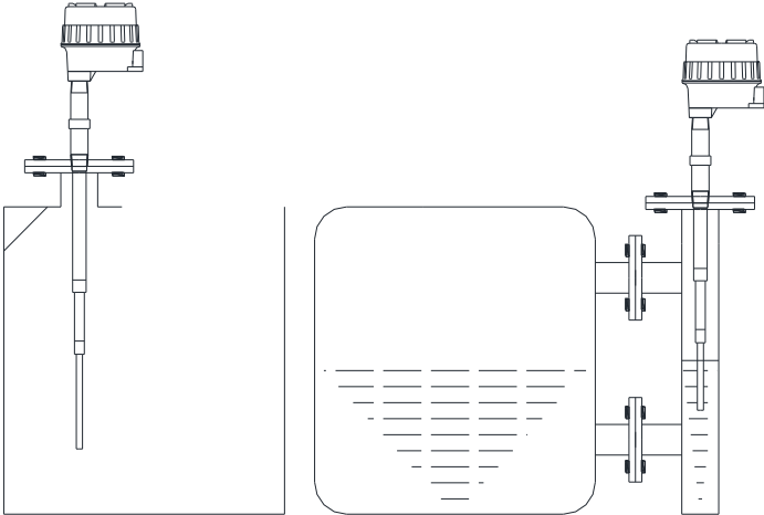
开放池的支架安装 外浮筒安装
