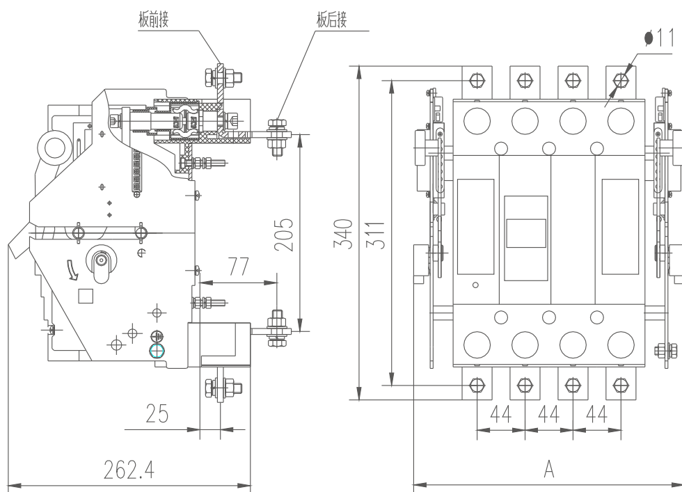
FTM2-400外形及安装尺寸
