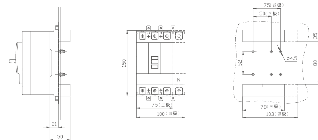
插入式板后接线（三极、四极）安装板开孔尺寸
