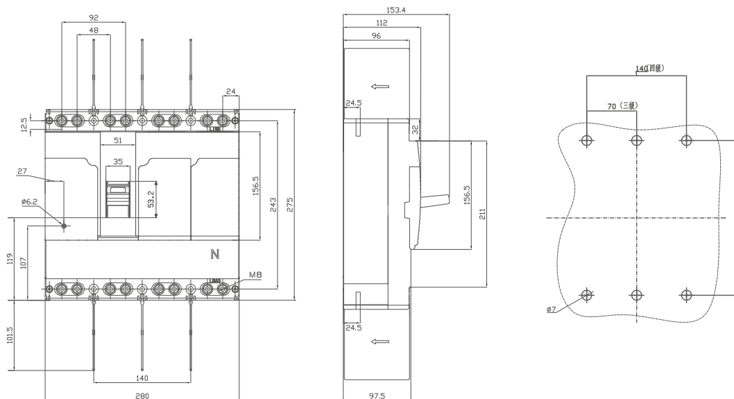
FTM2-800外形及安装尺寸
