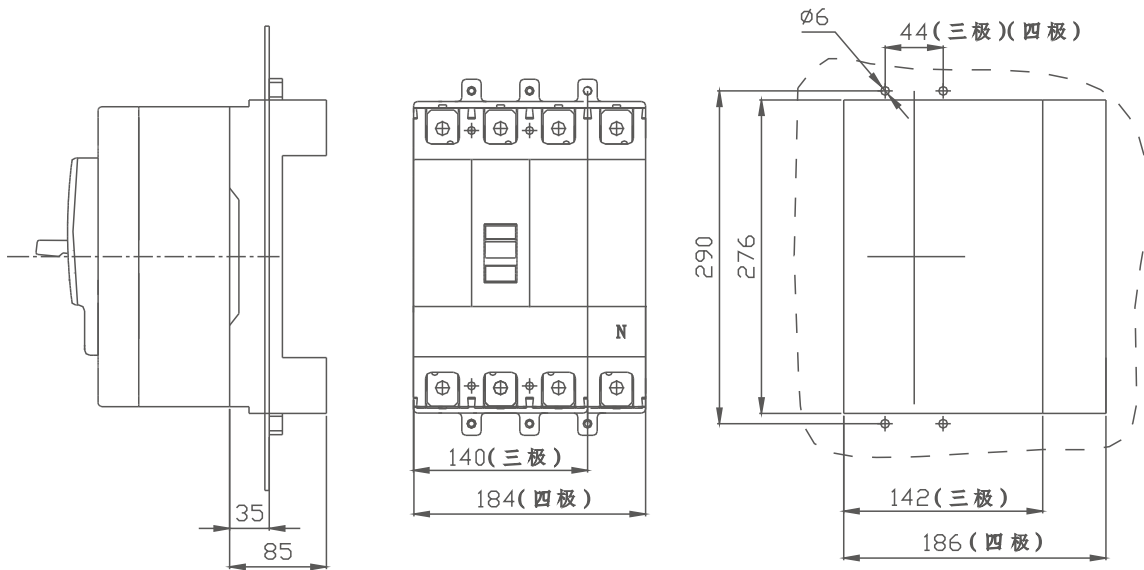
FTM2-400外形及安装尺寸
