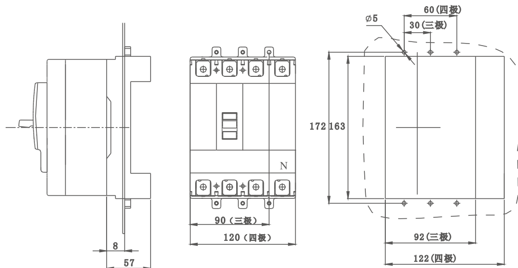
FTM2-160外形及安装尺寸
