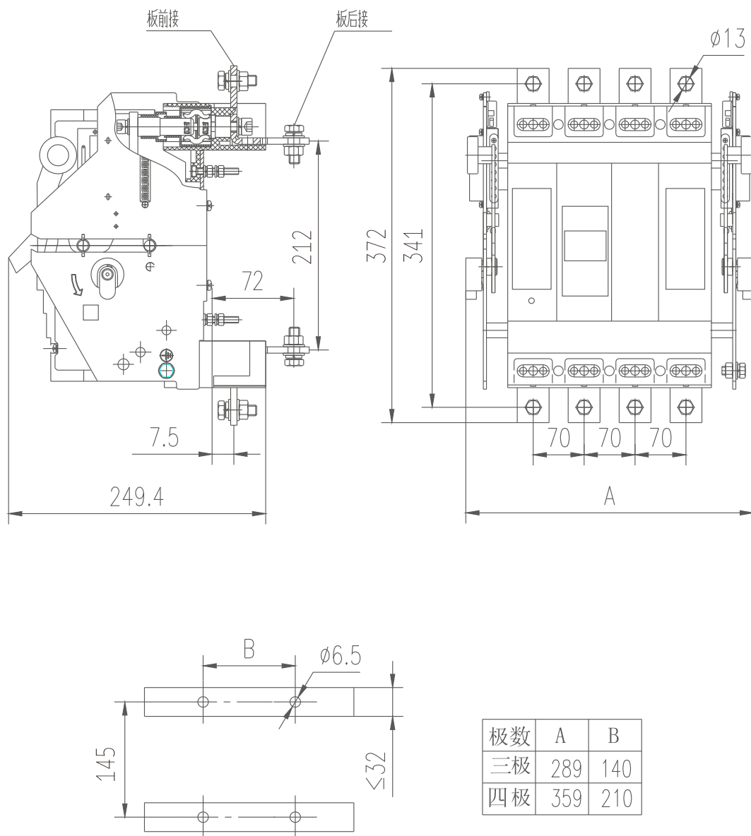
抽出式接线（三极、四极）安装板开孔尺寸
