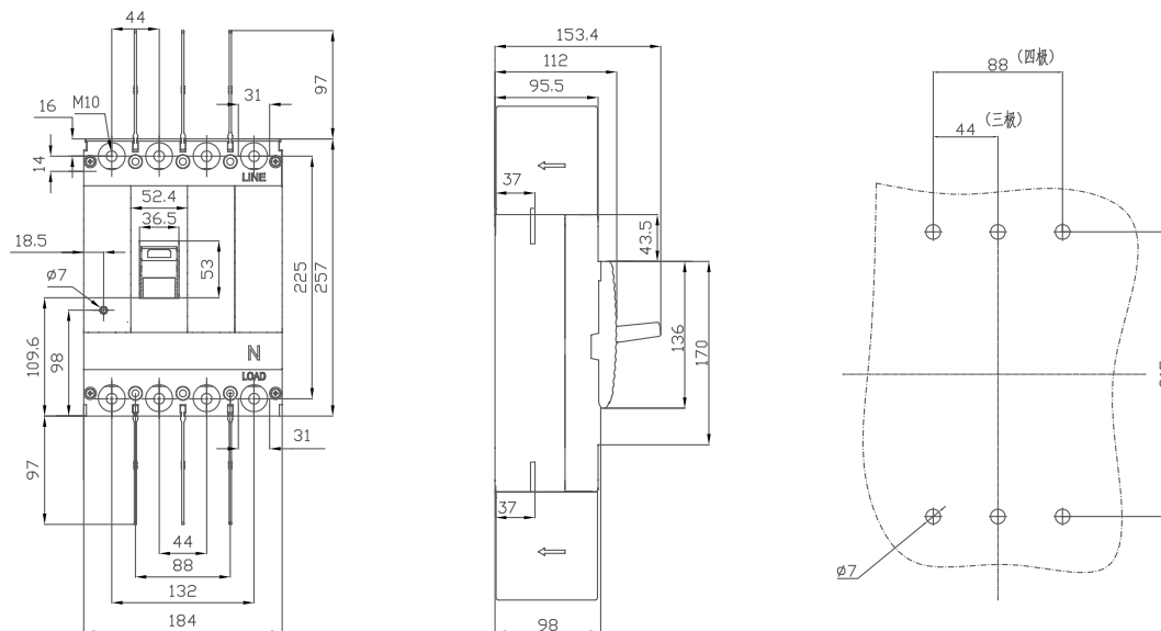
FTM2-400外形及安装尺寸
