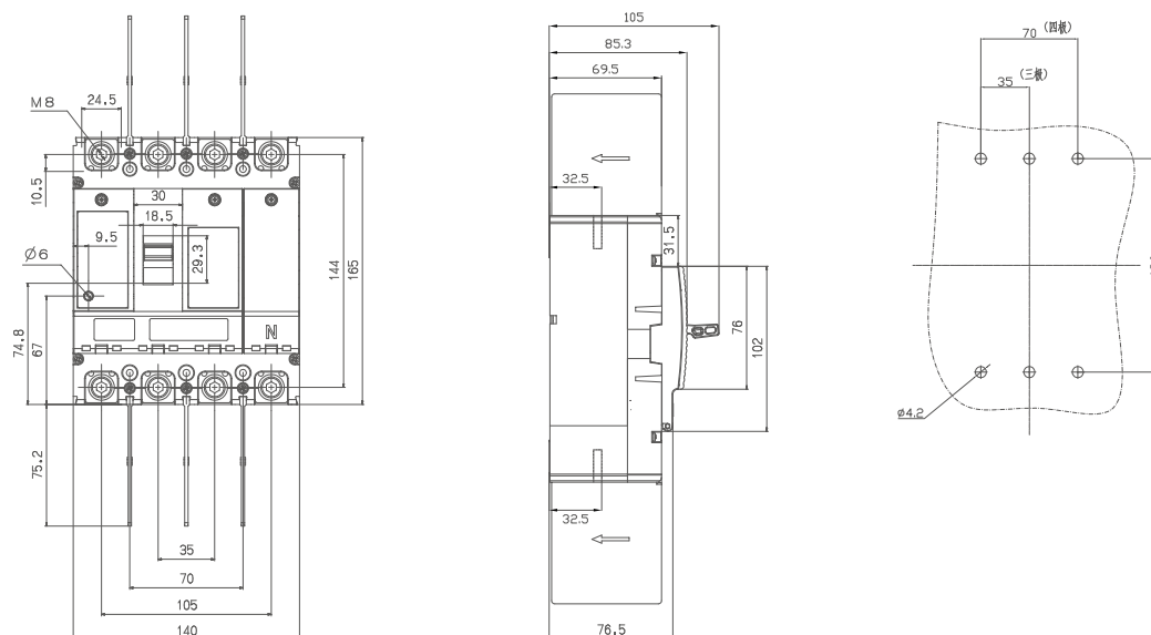
FTM2-250外形及安装尺寸
