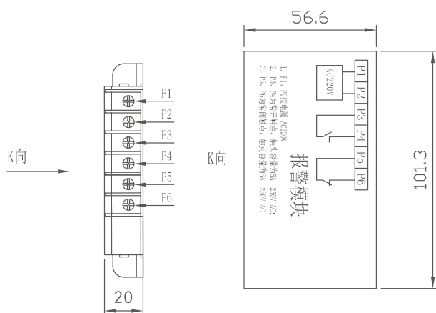
漏电报警模块尺寸图
