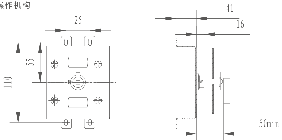
3) 中心式机构操作机构
