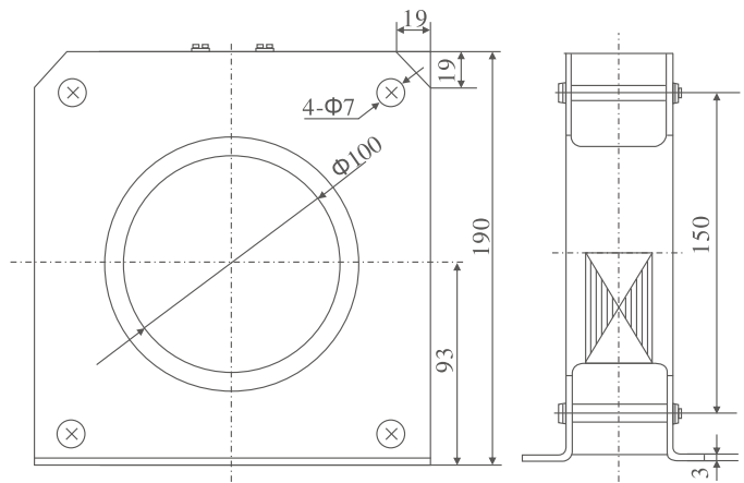
图9-6（ZT100地电流互感器）
