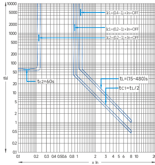
图7 负载监控方式二
