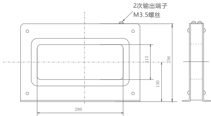
图9-7 ZCT1漏电互感器
