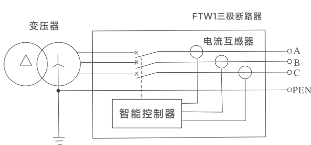
图9-1 3PT型 差值型接地故障保护，信号只取三相 电流的矢量和（三相不平衡）
