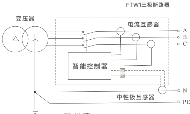
(3P+N) T型 外接中性极互感器 差值型接地故障保护，信号只取 三相电流及N相电流的矢量和
