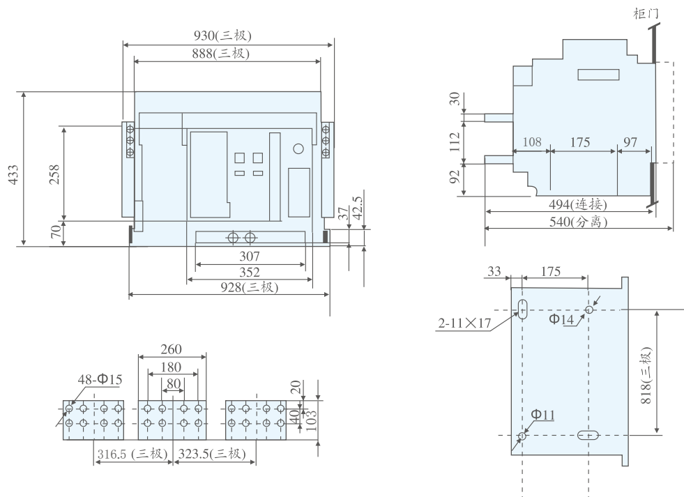
图11-8 抽屉式断路器安装尺寸及外形尺寸 (FTW1-6300/3, In=6300A)
