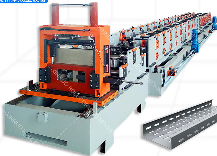
■ 电缆桥架成型设备
