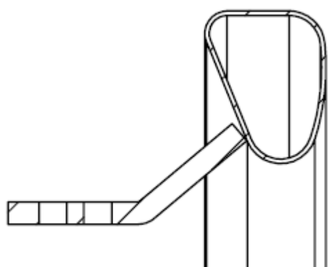
横截面
