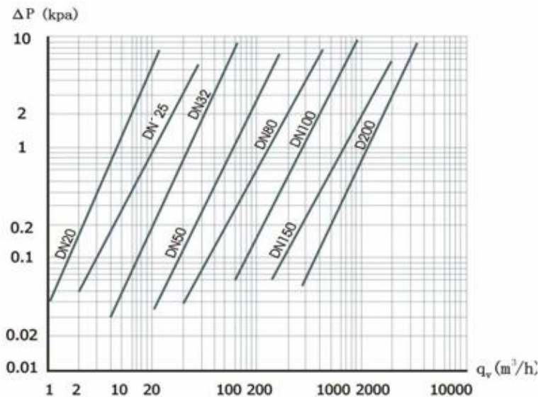
压力损失曲线
