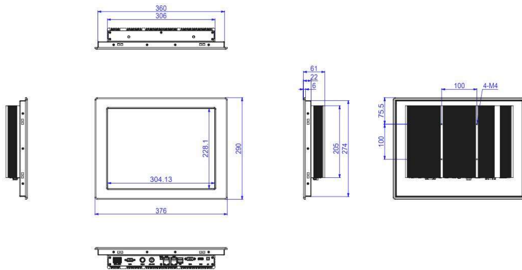
J1900 电阻触摸尺寸图
