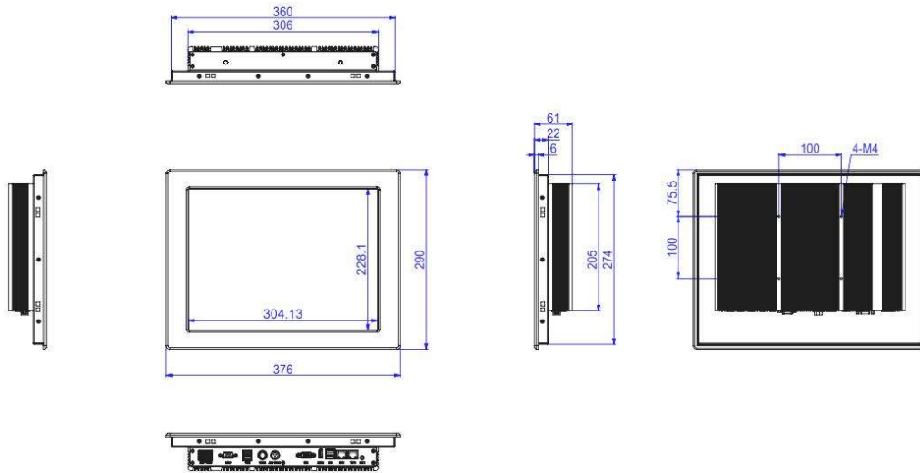
i5-6200U 电阻触摸尺寸图
