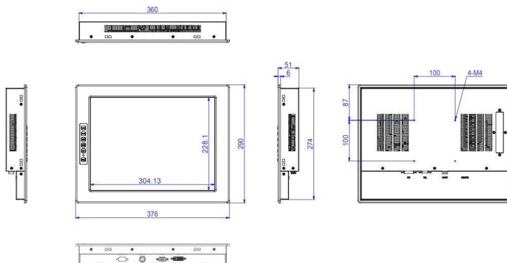
电阻触摸及无触摸尺寸图
