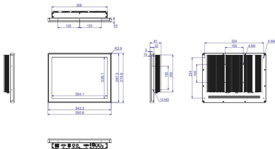
i5-6200U 电容触摸尺寸图
