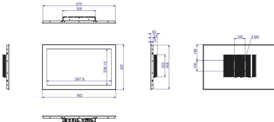
i5-6200U 电容触摸尺寸图
