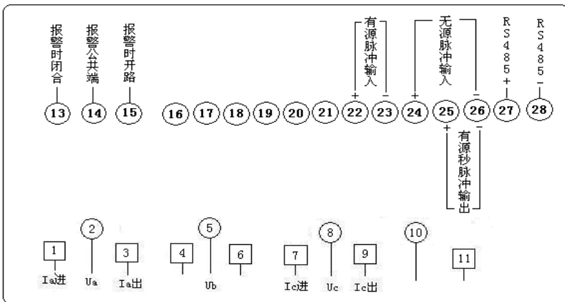
JSY-3BS接线图
