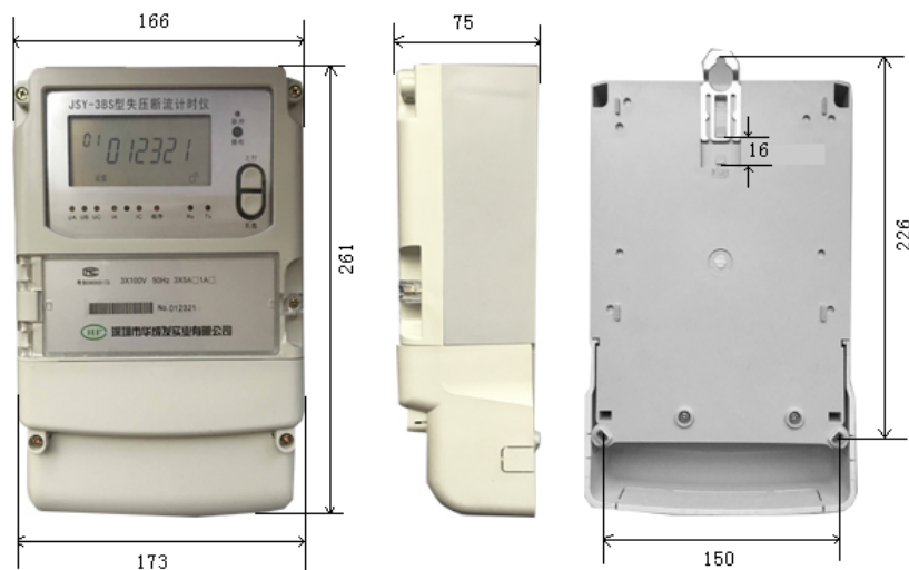
图三 安装尺寸图
