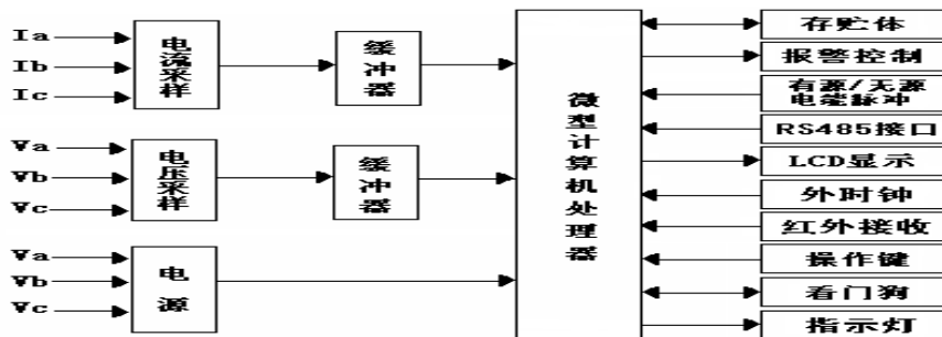
图一 工作原理框图
