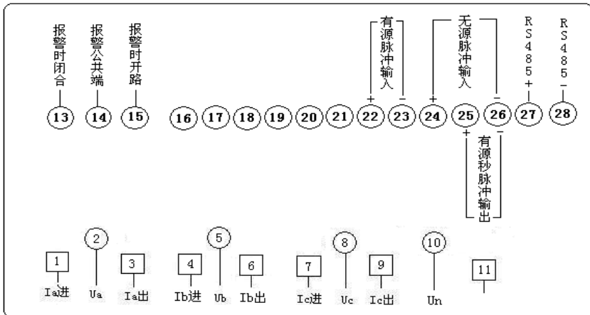
JSY-3BT接线图
