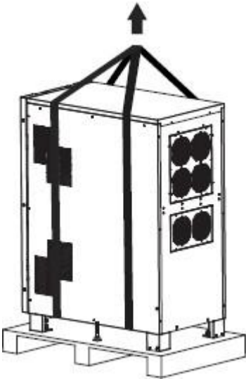
移除外箱及包材
