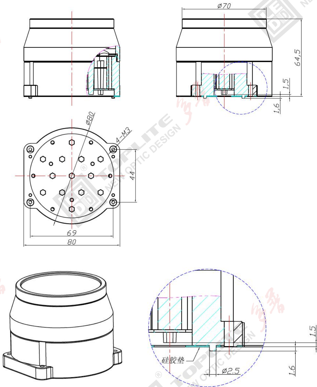
图 2: MATGOBO1360 系列聚光镜头机械尺寸
