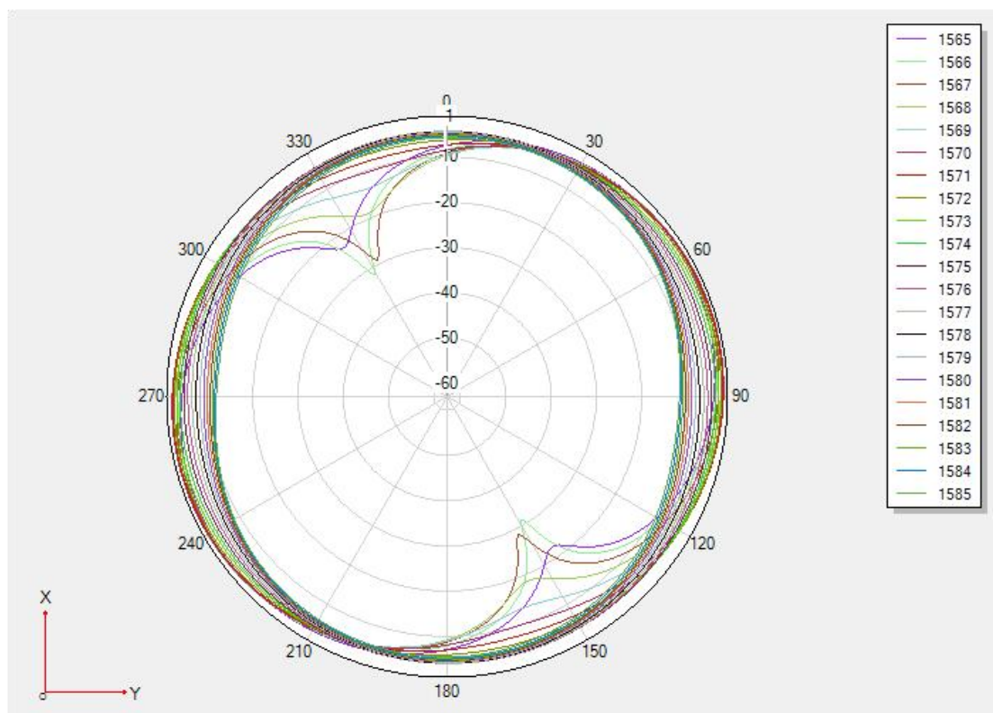
图 2 天线轴比
