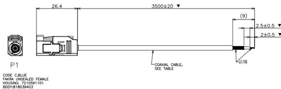
图 4 线材结构
