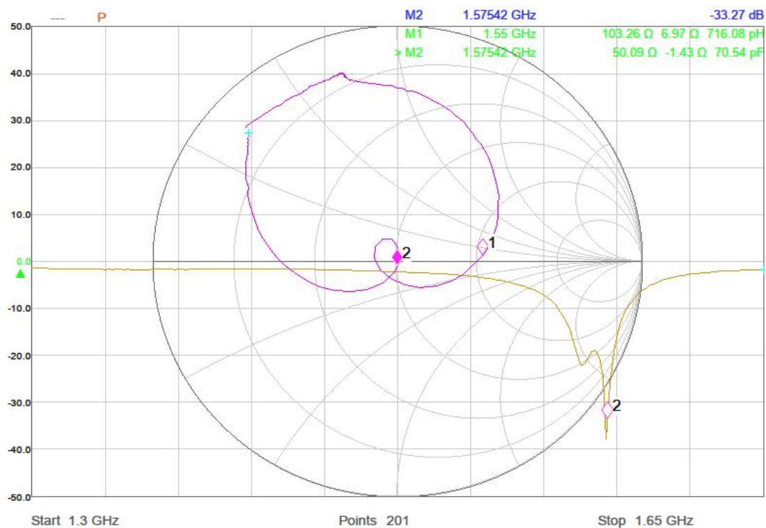
图 1 天线 S11
