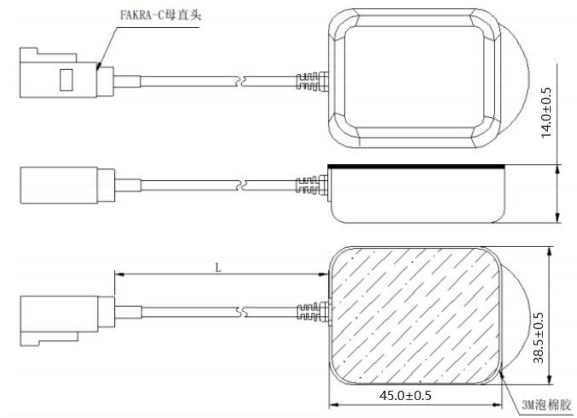
图 3 产品结构
