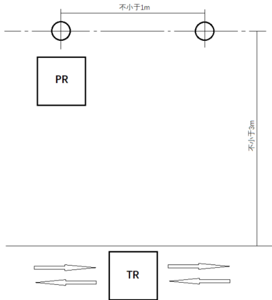
图 1 球、机器人的相对位置要求
