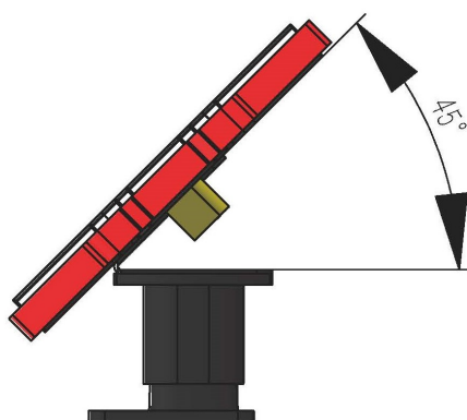
图 3-4(1) 45 度角安装生命柱
