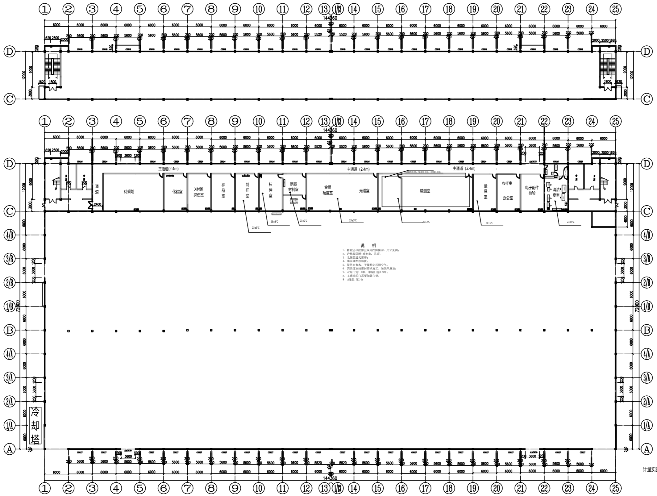
底层平面图
