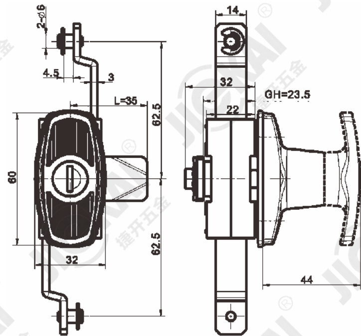
齿条连动型 Linkage for rack type
