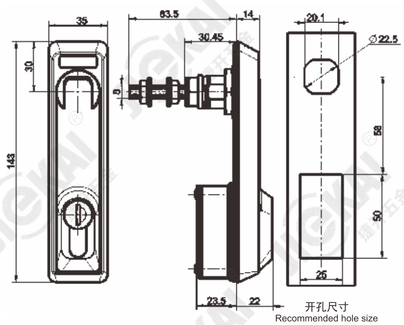
规格型号 Specifications PM208-3K2-M2
