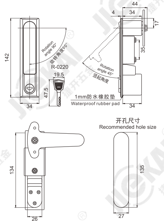
规格型号 Specifications PM499-1S1-G
