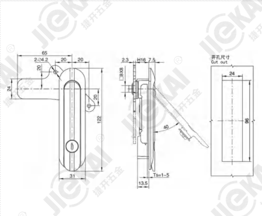
规格型号 Specifications PM252-1K1-E5
