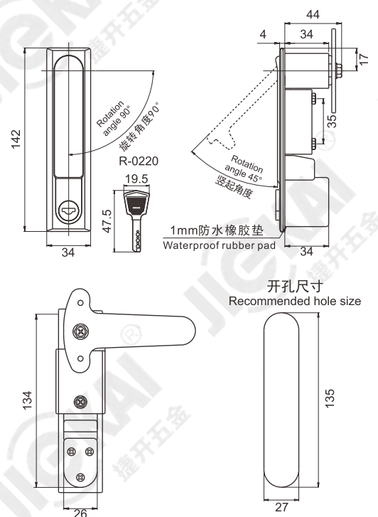
规格型号 Specifications PM490-1S1-B
