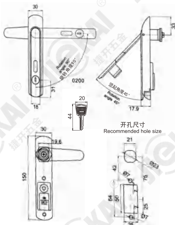
规格型号 Specifications PM4501-1K1-S
