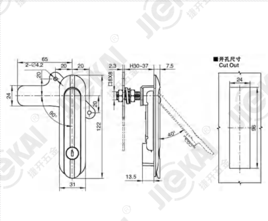
规格型号 Specifications PM253-1K2-E5
