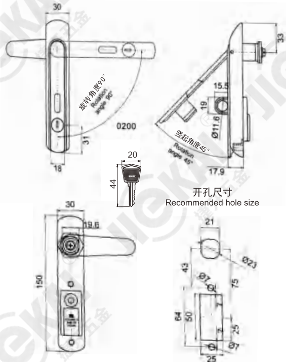
规格型号 Specifications PM4502-1S1-S
