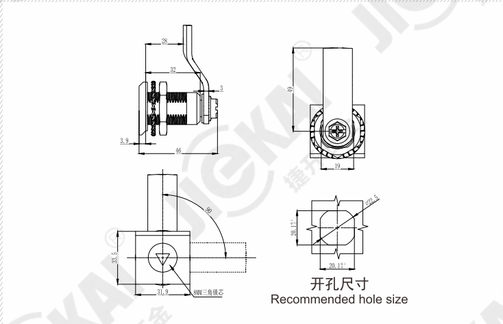
A型 工程图 Engineering drawing
