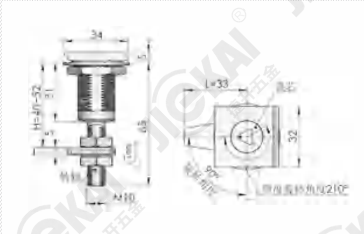
B型 工程图 Engineering drawing
