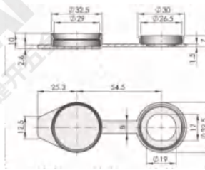
锁头防水盖(选配) Waterproof cap(optional)
