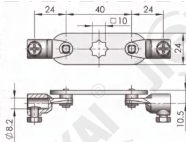
选配钢栓 Optional steel bolt
