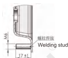
选用面板 Optional panel
