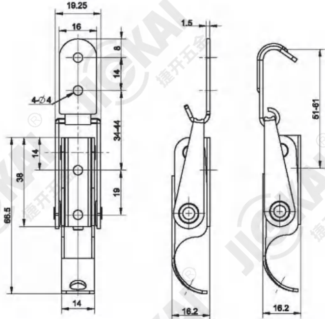
标准拉扣 Standard pull clasp SD909-3NXX
