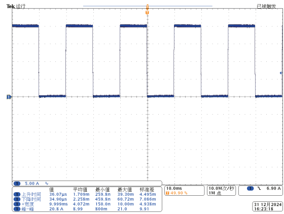
正脉冲波形
