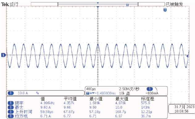
5kHz频率带宽波形
