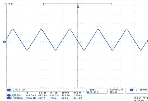
500Hz频率带宽波形
